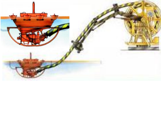
海上油污回收與輸送獨立整合系統 功能組裝示意 Hiwax Skimmer (Klemfare, USA)
