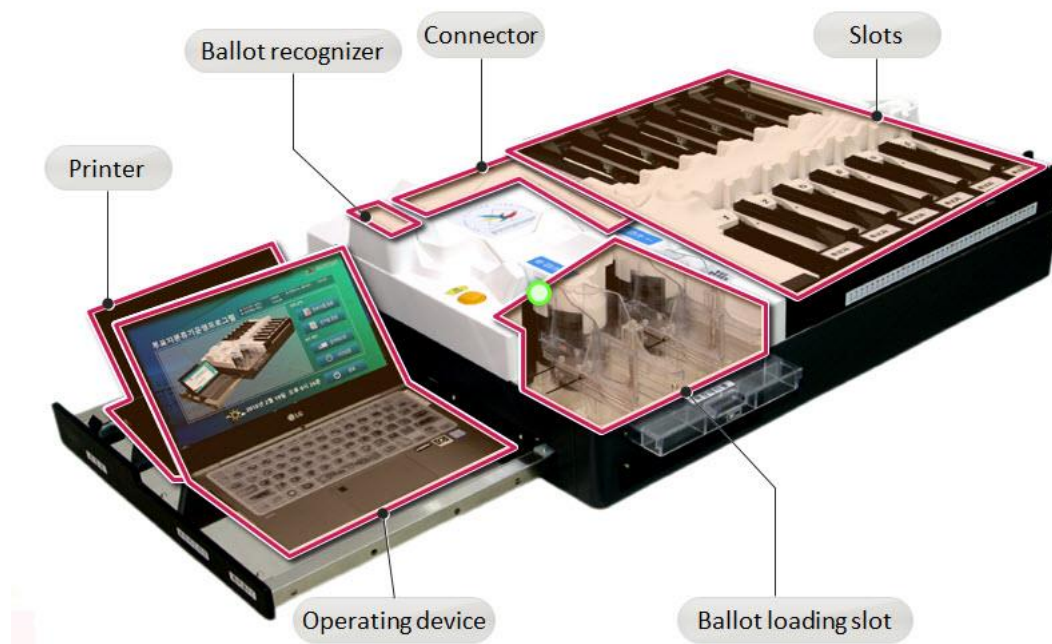
韓國開票作業使用之選票分類機
