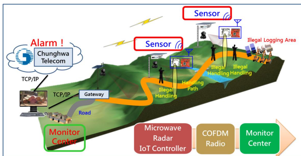
圖 3：應用物聯網及資通技術監控非法盜伐之系統架設示意圖
