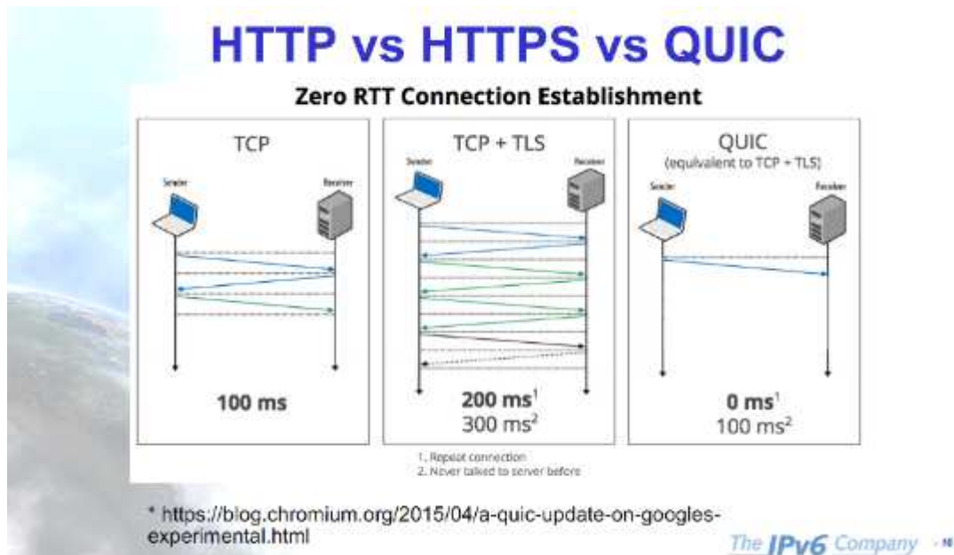
圖10、HTTP 與 QUIC 間的比較
