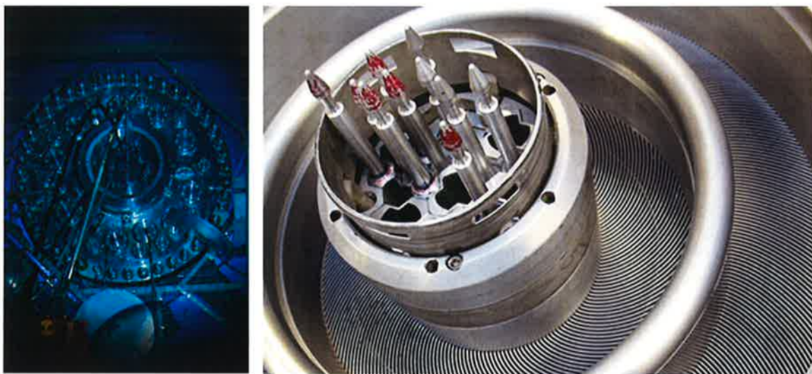
圖 14 高中子通量同位素反應器 (High Flux Isotope Reactor, HFIR)
