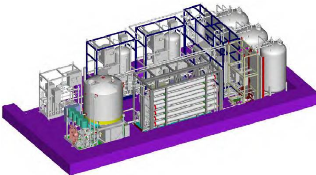
圖十、River Bend 核能電廠(位於路易斯安那州)之廢液處理系統
