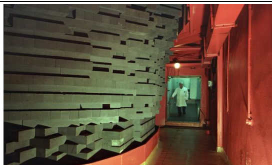
\Phi -1 反應器底部石墨堆
