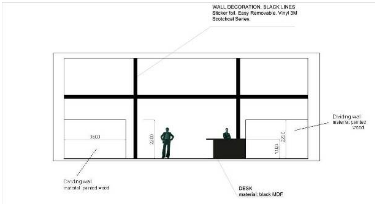
【圖 19】展館立面設計圖
