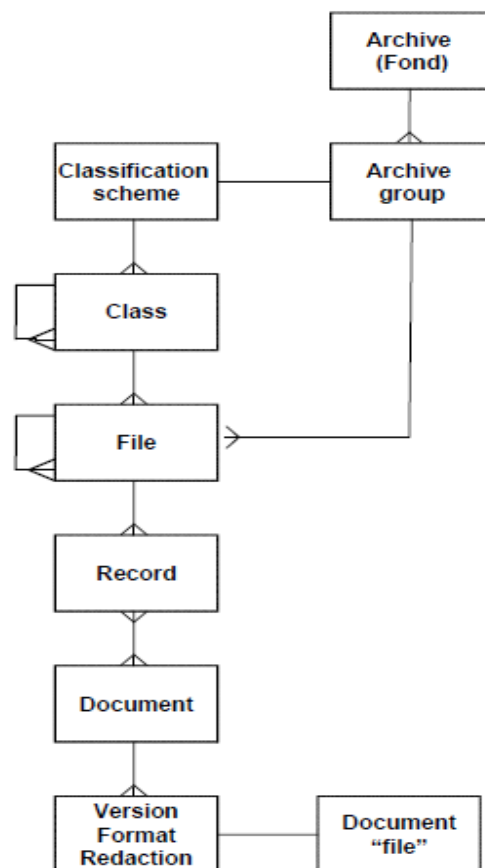
圖7 諾亞標準version 5電子檔案標準邏輯結構
