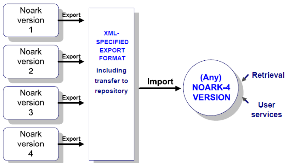
圖6 諾亞標準version 4資料轉置及移轉流程
