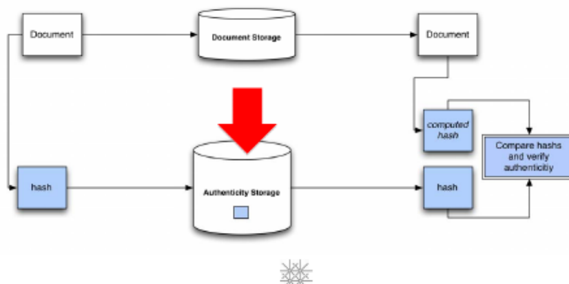
圖2 數位檔案真實性—雜湊值問題圖示
