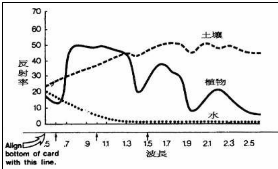
圖 2-3 土壤、植物及水體之光譜反射特性曲線
