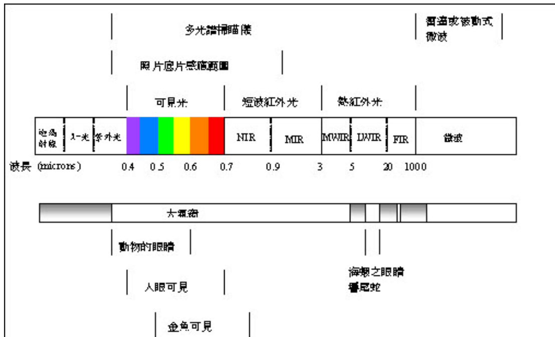
圖 2-2 電磁波之光譜圖
