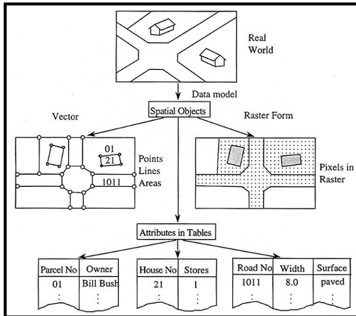
圖 2-4 地理資料-圖形資料與屬性資料
