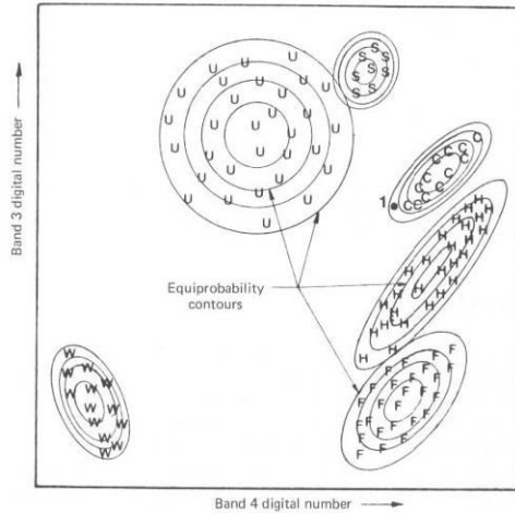
圖 2-17 最大概似法之決策示意圖
