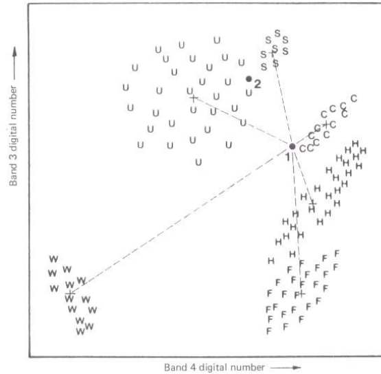
圖 2-13 最小距離法之決策示意圖
