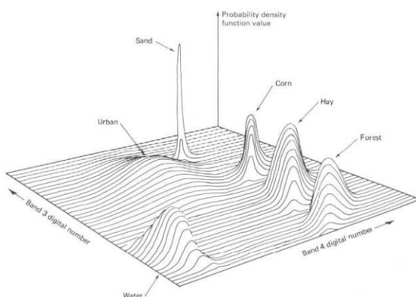
圖 2-16 訓練樣區點的統計機率圖
