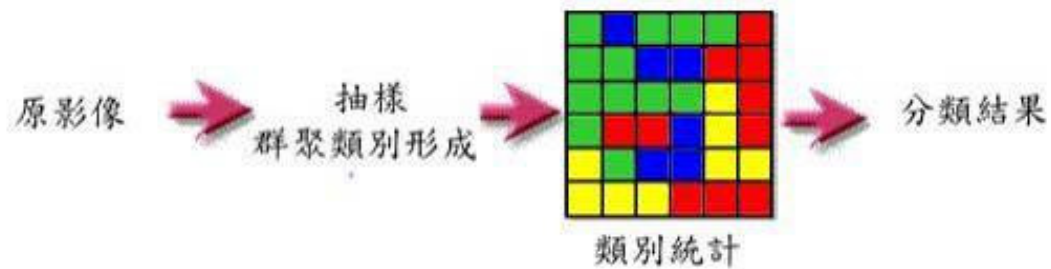
圖 2-18 非監督式分類法
