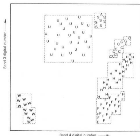
圖 2-15 平行六面體法(階梯狀)之決策示意圖
