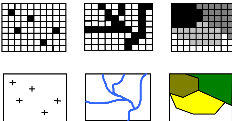
圖 2-5 向量資料與網格式資料的點、線、面模型
