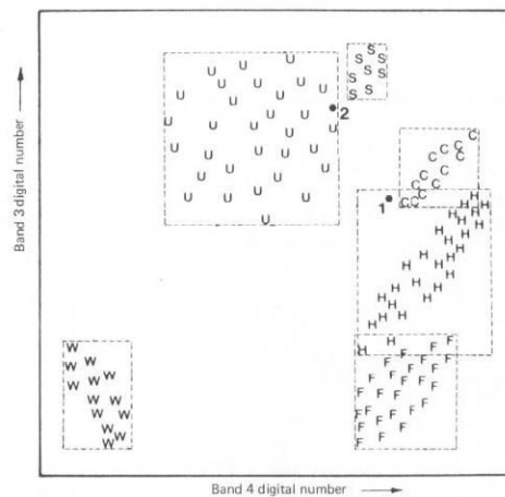
圖 2-14 平行六面體法之決策示意圖
