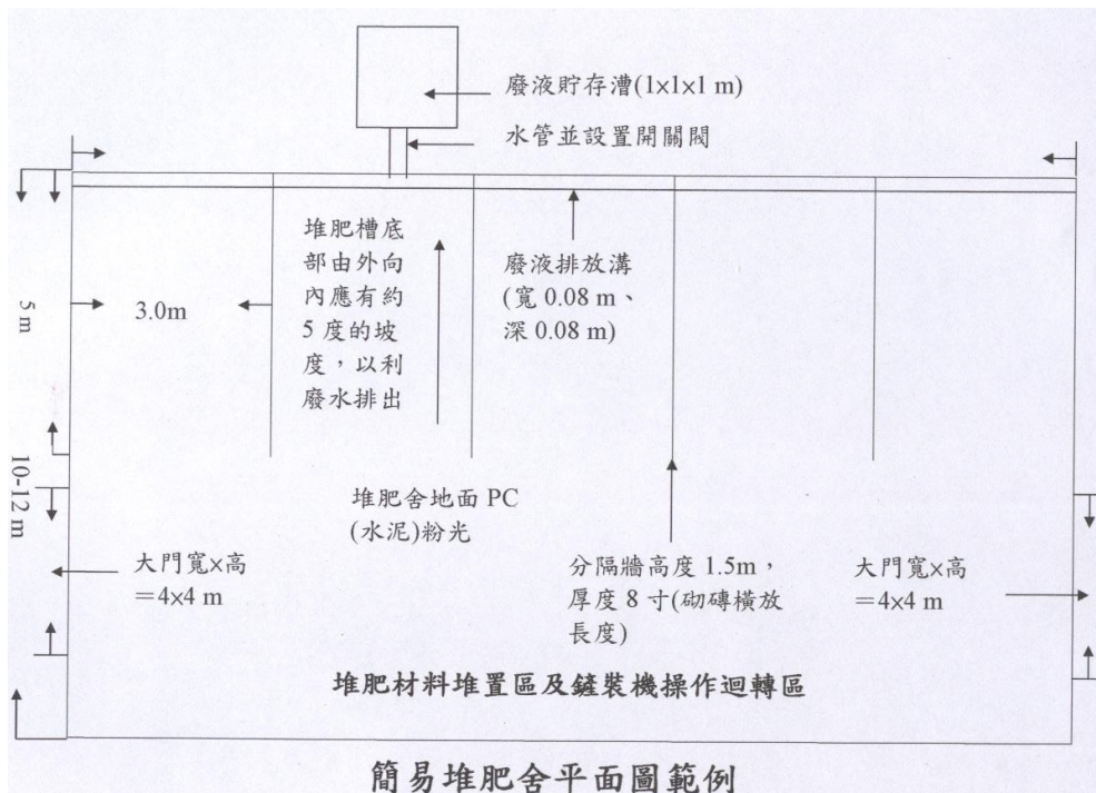
圖 15. 簡易堆肥舍平面圖
