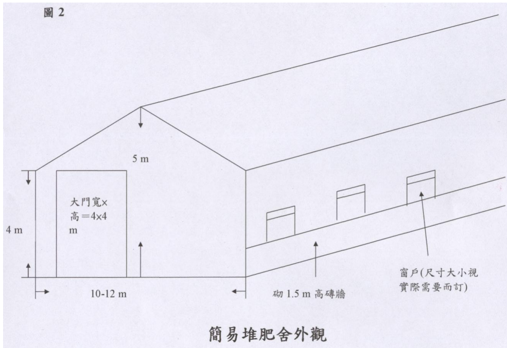
圖 14. 簡易堆肥舍外觀
