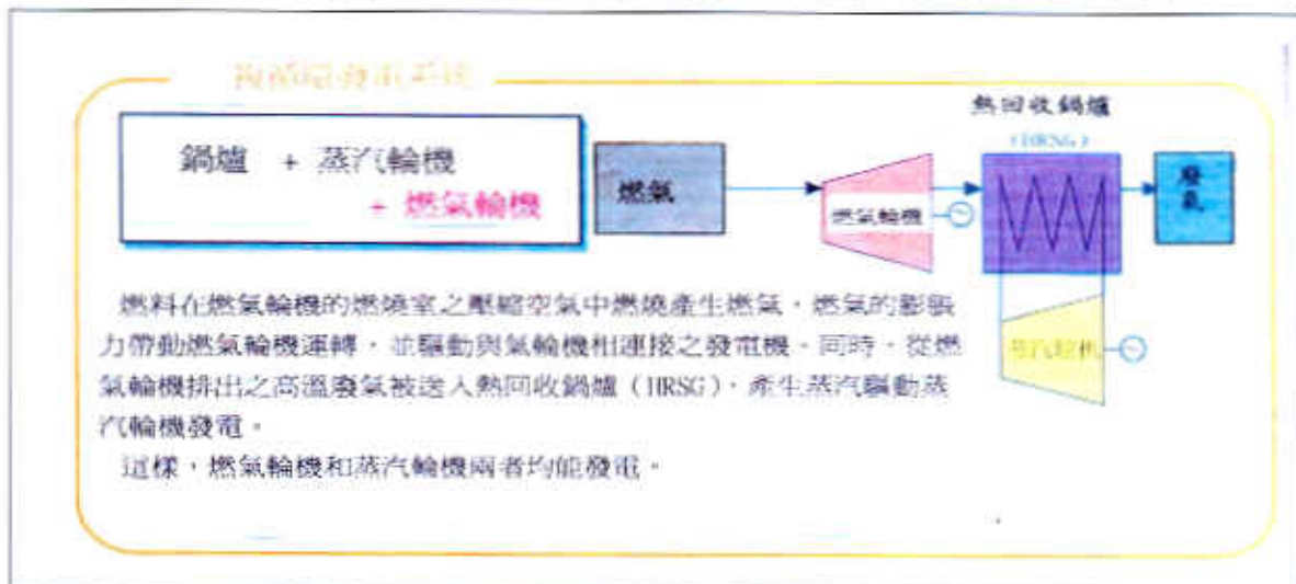
圖 17 複循環發電系統圖
