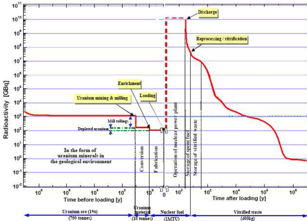
圖六 核燃料從開採、使用及棄置成為廢棄物活度變化衰減圖
