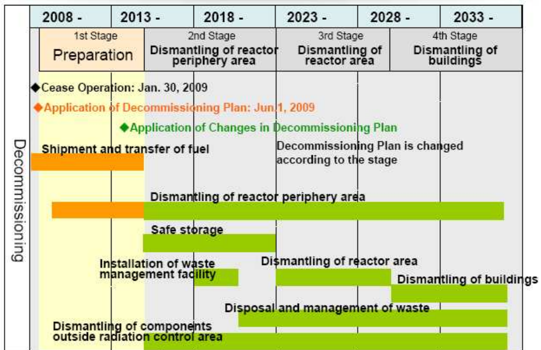
圖二 濱崗核能電廠 1、2 號機除役步驟之時程規劃
