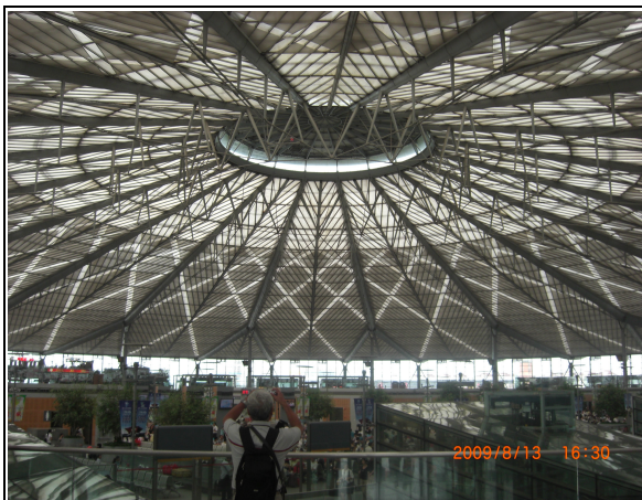
圖 65：上海南站高架車站採圓型造形之站體，直徑 267 公尺，挑高 42 公尺
