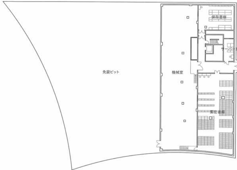
B1F平面図
