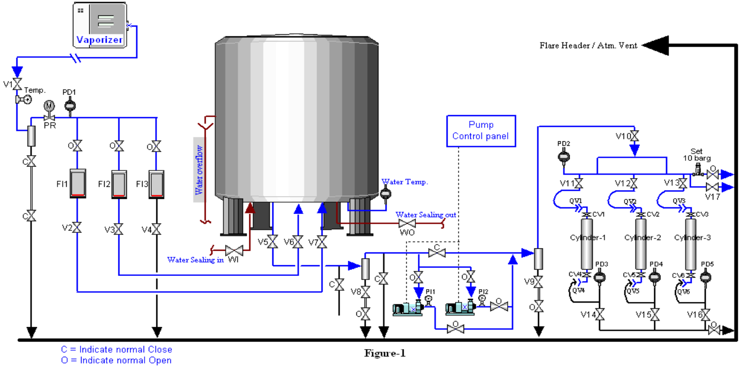
圖-1 取樣系統示意圖
