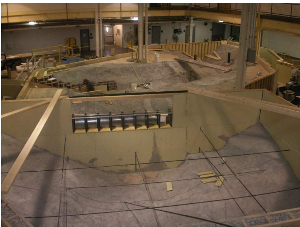
照片六 美國墾務局水資源研究試驗室(WRRL)以木材製作模型
