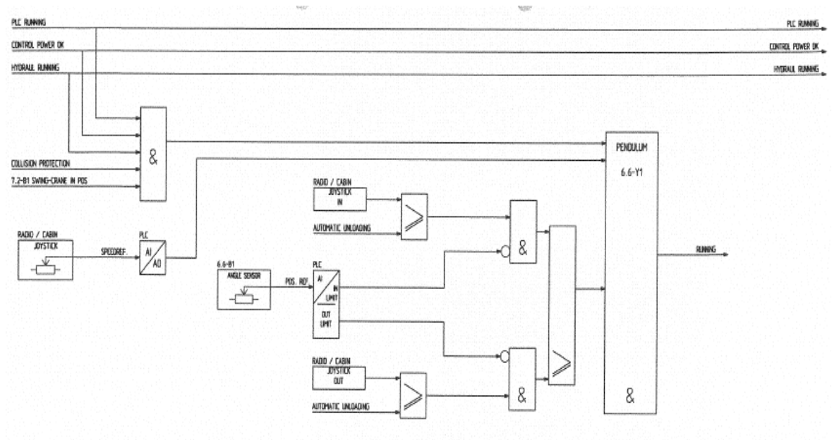
圖 10 擺錘(Pendulum)邏輯圖
