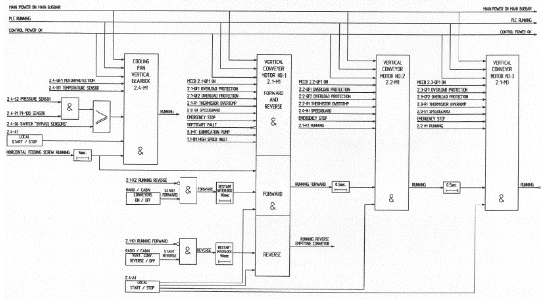
圖 5 垂直輸送帶(Verticle conveyor)
