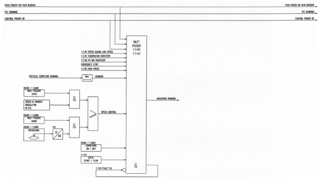
圖 6 進料器(Inlet feeder)
