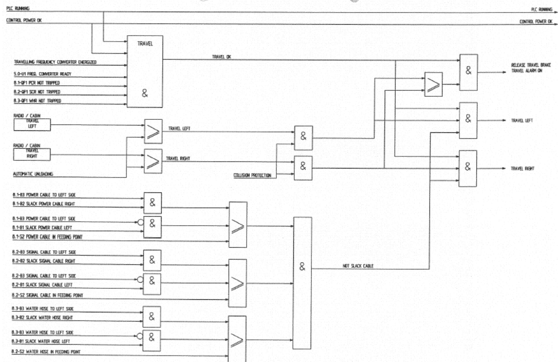
圖 11 移動(traveling)邏輯圖
