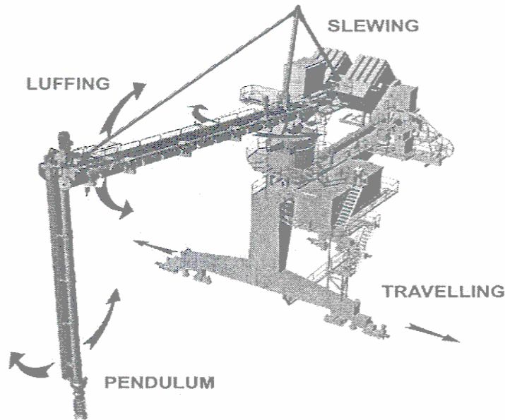
圖 7 卸煤機運動系統(Motion system)示意圖
