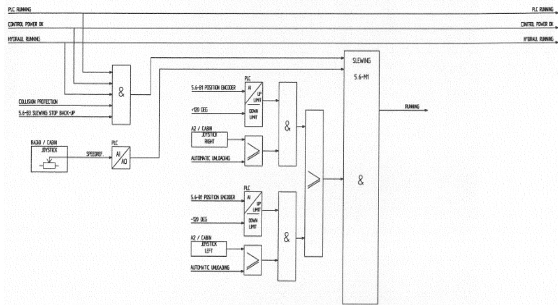
圖 8 轉動(Slewing)邏輯圖
