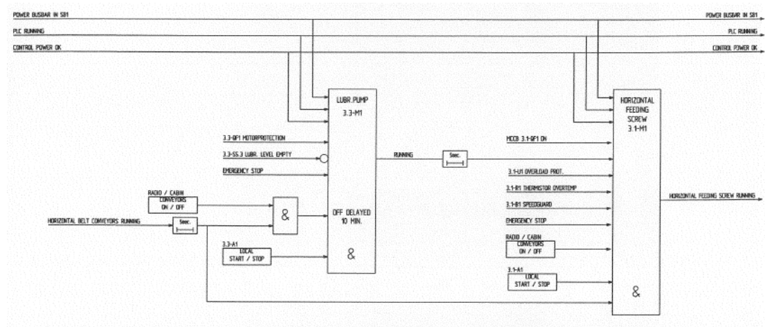
圖 4 水平進料螺旋輸送帶 Horizontal feeding screw
