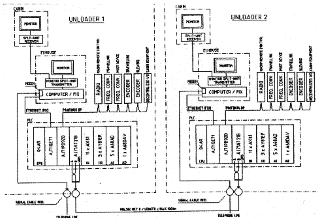
圖 1 卸煤機控制系統架構圖
