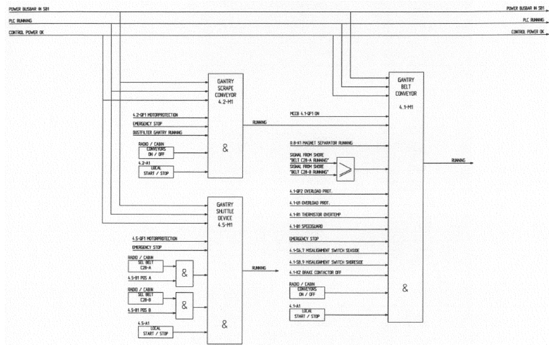
圖 2 臺架皮帶機(Gantry belt conveyor)邏輯圖
