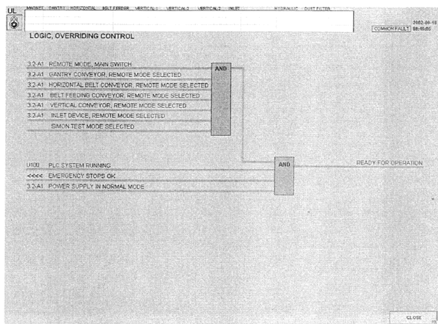
如圖 16 越權控制(OVERRIDING CONTROL)
