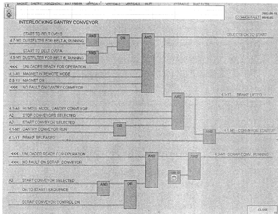
圖 19 物件互鎖(Object interlocking)
