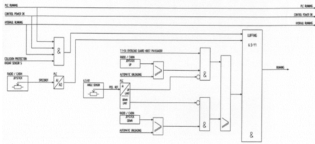
圖 9 上下擺動(Luffing)邏輯圖
