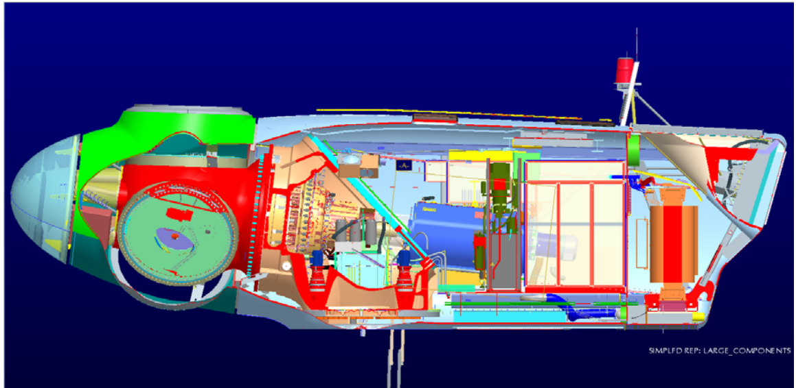
Fig. 1 V90-3.0 MW Nacelle
