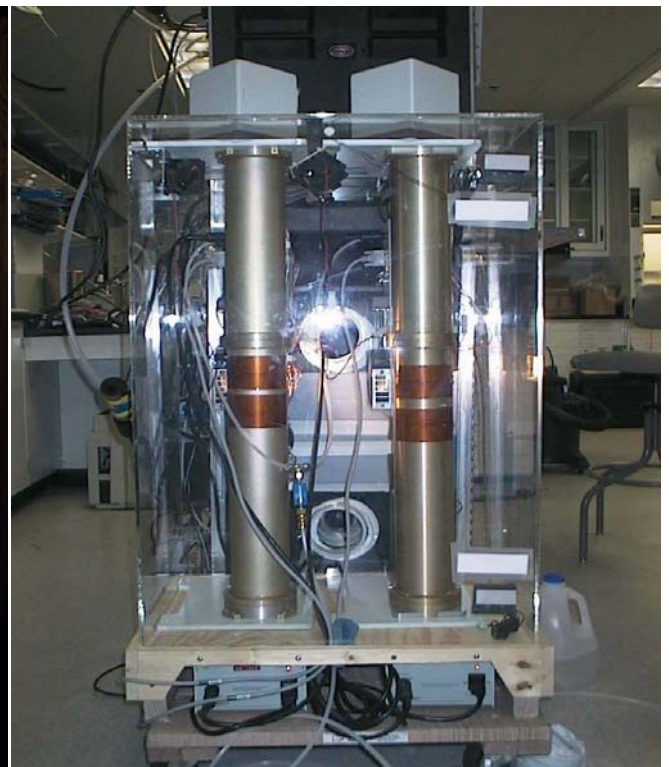
圖二、散光儀
