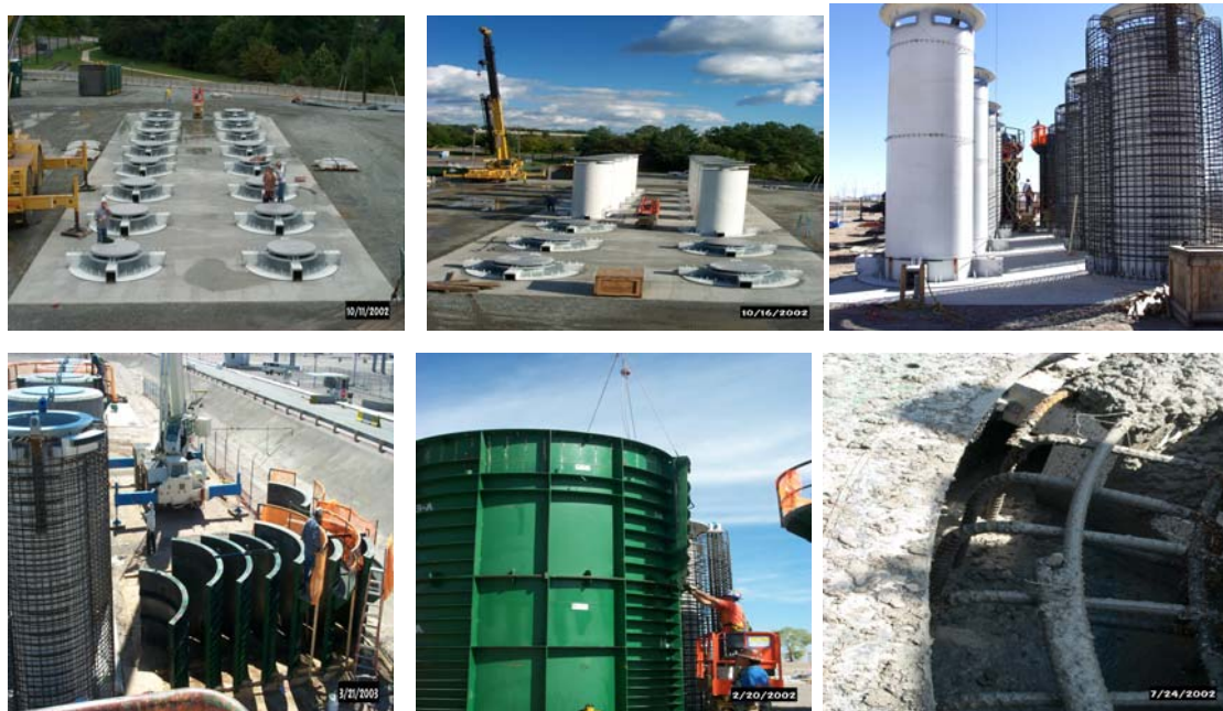
圖 7 混凝土護箱建造（對位契合、綁鋼筋、架設模具、灌漿澆置）
