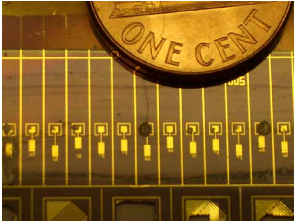
相片十五、鋅鈦酸鉛溶膠薄膜製成之微致動器元件
