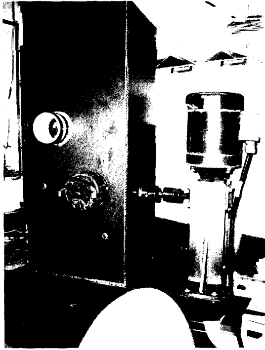
圖 6 魚卵與仔稚魚自動分離設備
