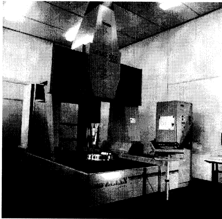
圖 2-22 輪軸組裝前檢驗
