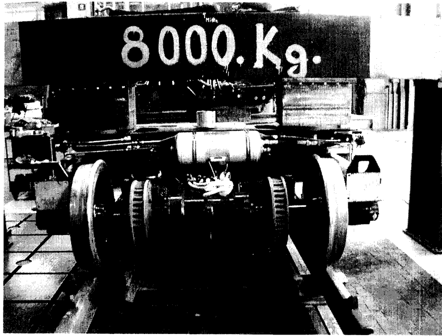
圖 2-48 轉向架總成靜負載檢驗
