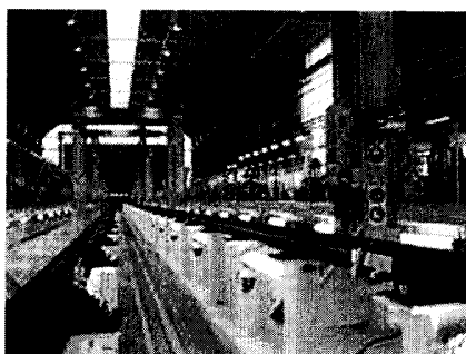
圖 2-27 靜態輪重量測系統(SWWS)
