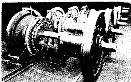
圖 2-16 GHH 輪軸成品
