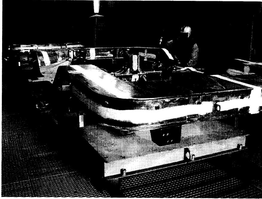
圖 2-42 轉向架表處前處理
