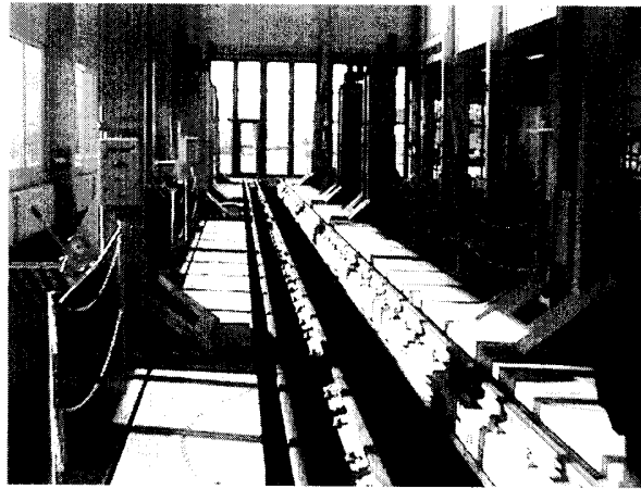
圖 2-12 車輛及轉向架升降機
