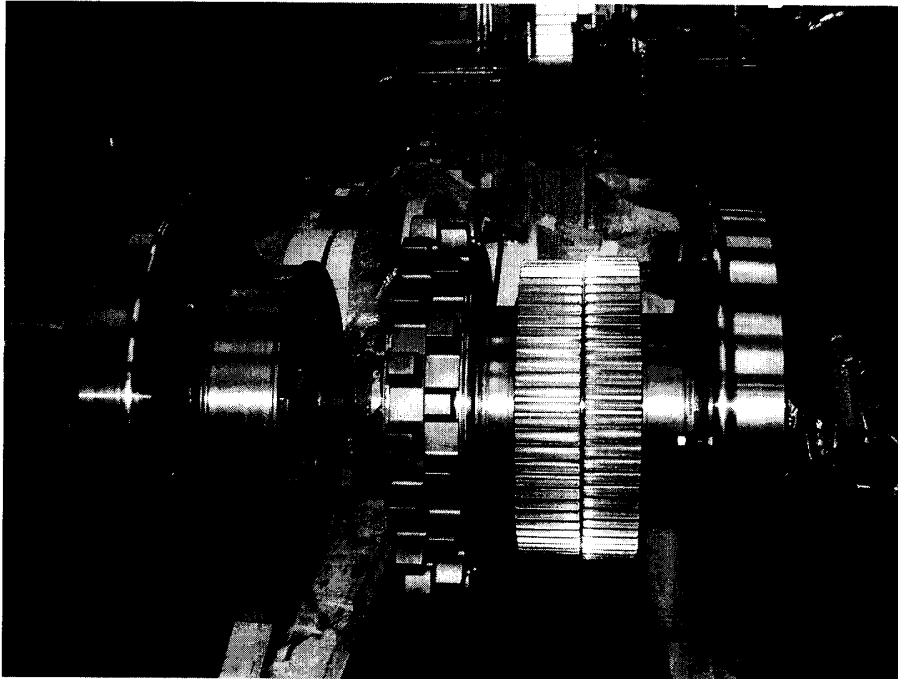
圖 2-37 瑞士登山火車驅動輪軸組
