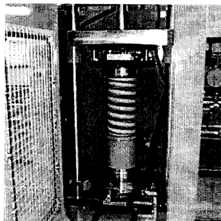
圖 2-23 螺旋彈簧靜態測試台
