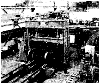
圖 2-25 簡易型全自動轉向架測試台
