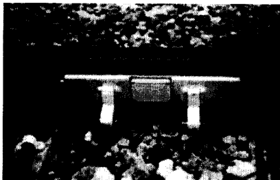
圖 2-26 靜態輪重量測系統(SWWS)
