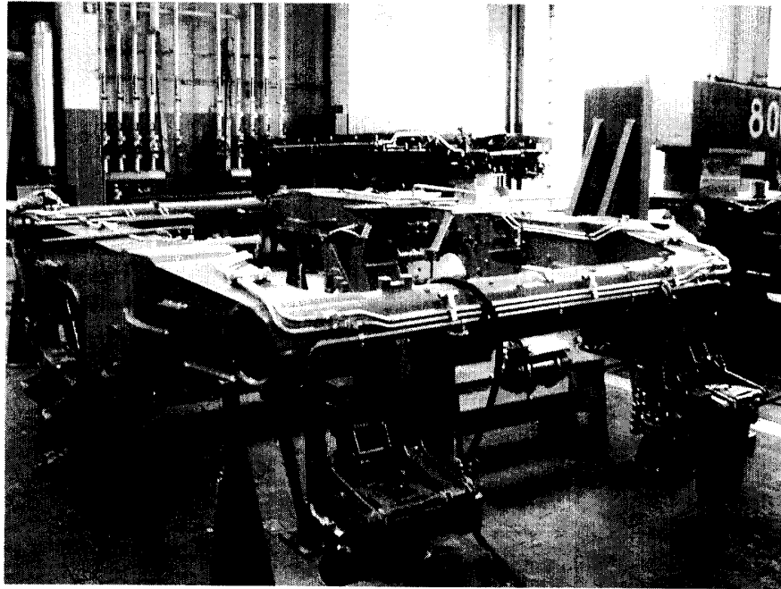
圖 2-43 轉向架管線安裝
