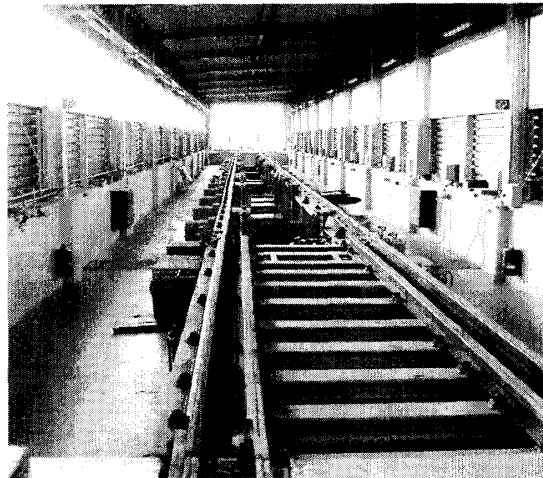
圖 2-10 靜態測試平台
