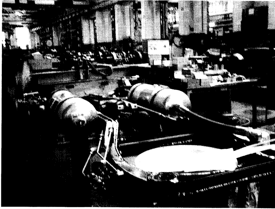
圖 2-44 轉向架承樑組裝現場工作狀況
