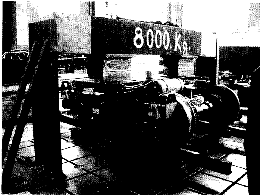
圖 2-49 轉向架總成靜負載檢驗
