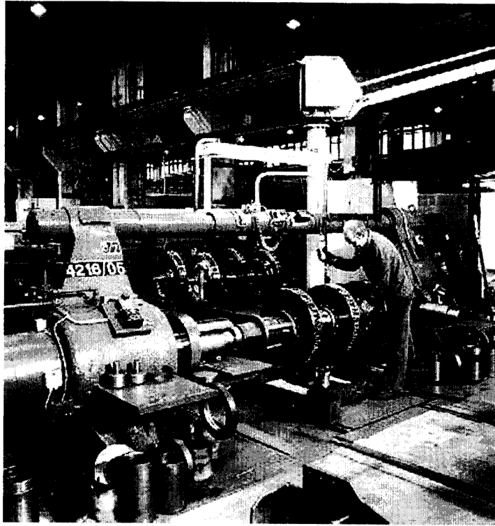
圖 2-21 剎車盤壓入輪軸過程
