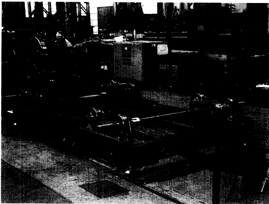
圖 2-47 轉向架總成輪軸滾轉測試台及工作溝
