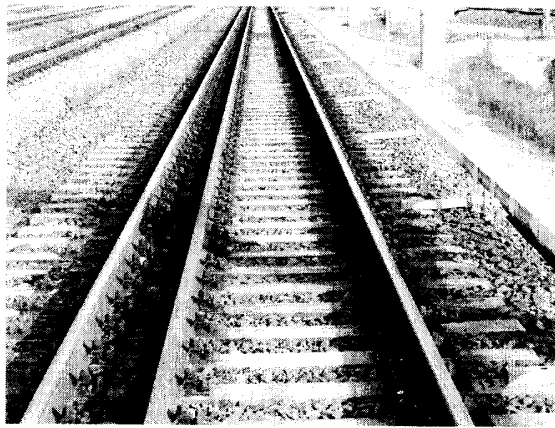
圖 2-13 標準軌與米軌複軌系統
