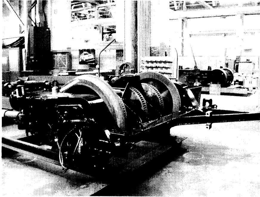
圖 2-50 單軸式轉向架成品
