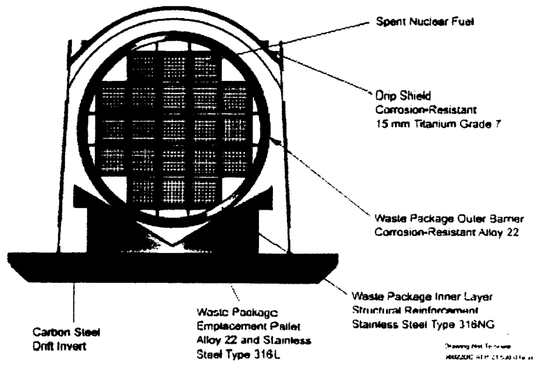
4-6 處置容器與基座之概要圖
