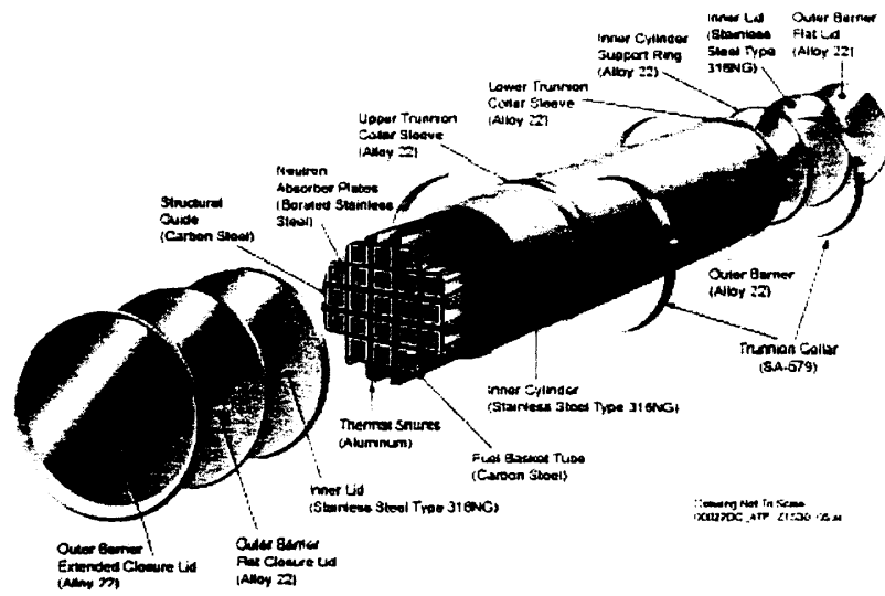
圖 4-1 21PWR 處置容器圖
