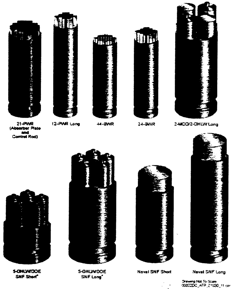
圖 4-3 廢料體與處置容器之設計圖
