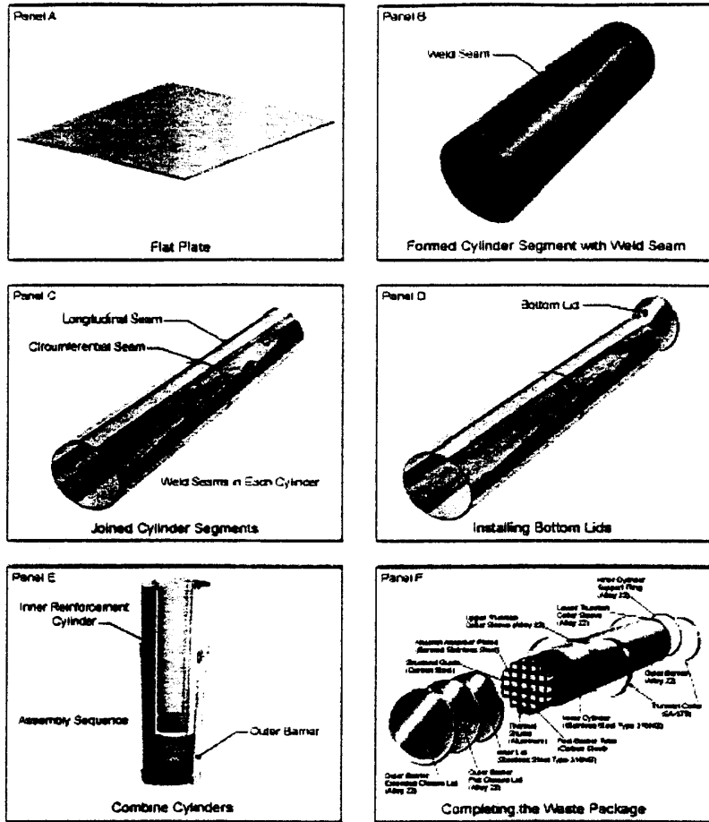
圖 4-7 處置容器之製程
