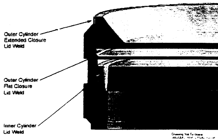
圖 4-8 處置容器之密封焊接圖示
