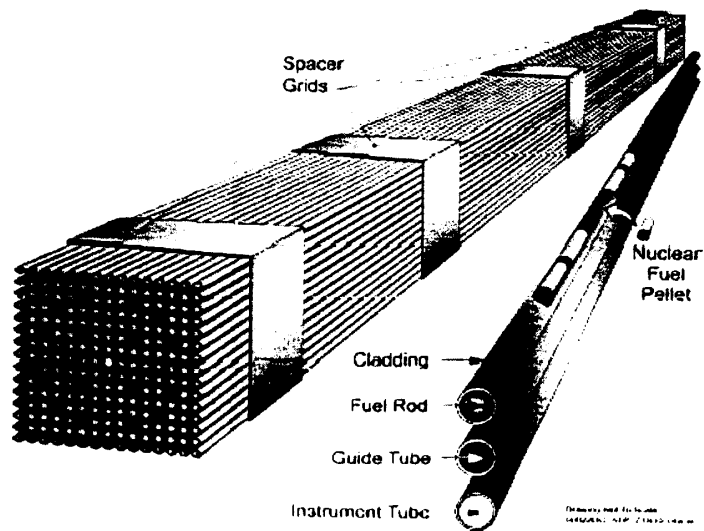
圖 4-4 典型之 PWR 燃料元件圖例
