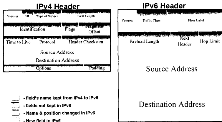
圖 1：IPv4 與 IPv6 表頭格式
