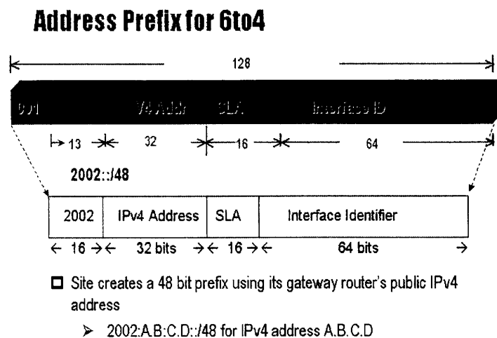
圖 19：6 to 4 Address Format
