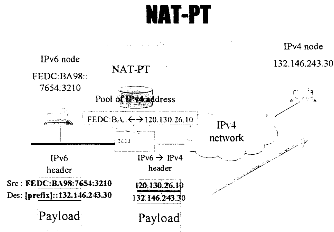
圖 22：NAT-PT 示意圖
