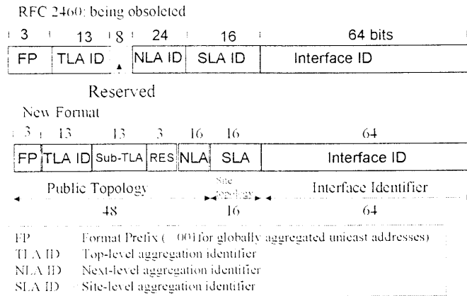
圖 4：IPv6 位址分級架構
