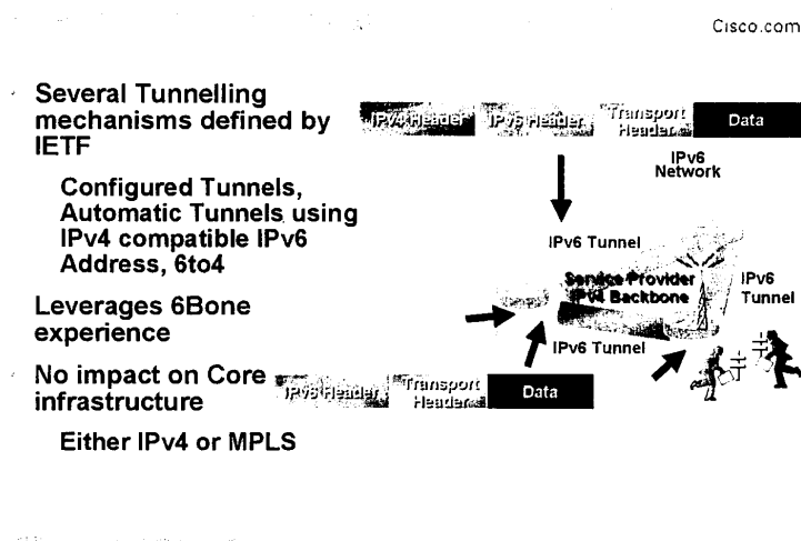
圖 7：IPv6 over IPv4 Tunnel
