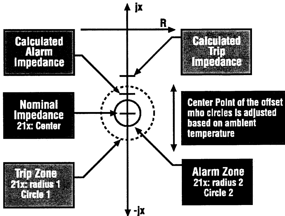
圖八：阻抗法電容器阻保護特性
