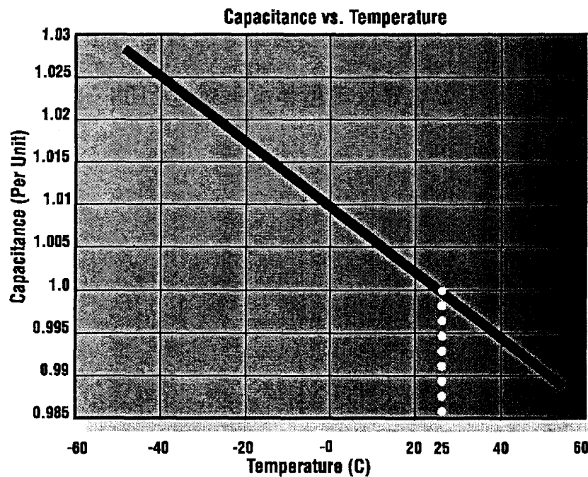
圖七：電容值與溫度的關係
