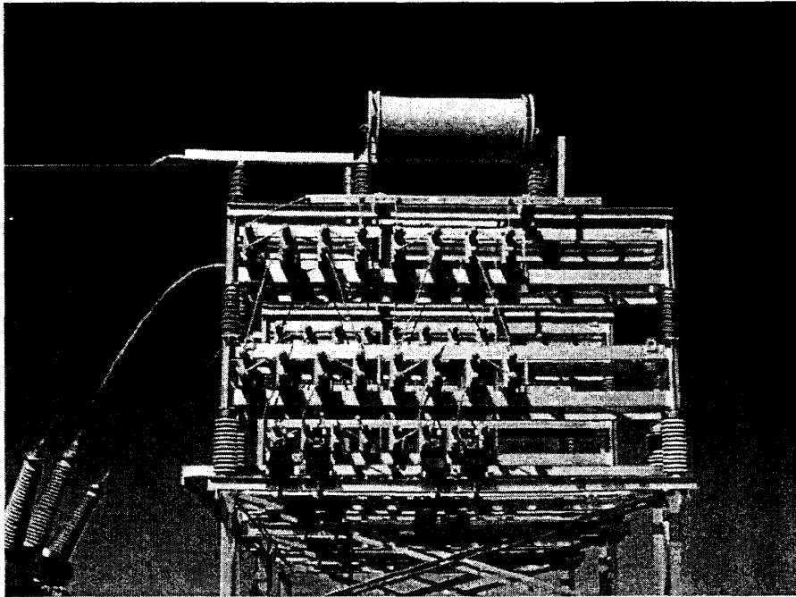
圖五：R相照片
