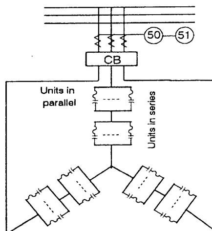
圖二：Shunt Capacitor Bank
