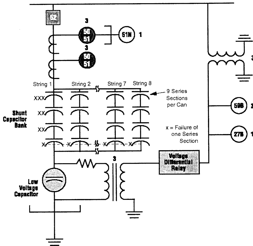
圖十：分散式故障 和 累積式故障
