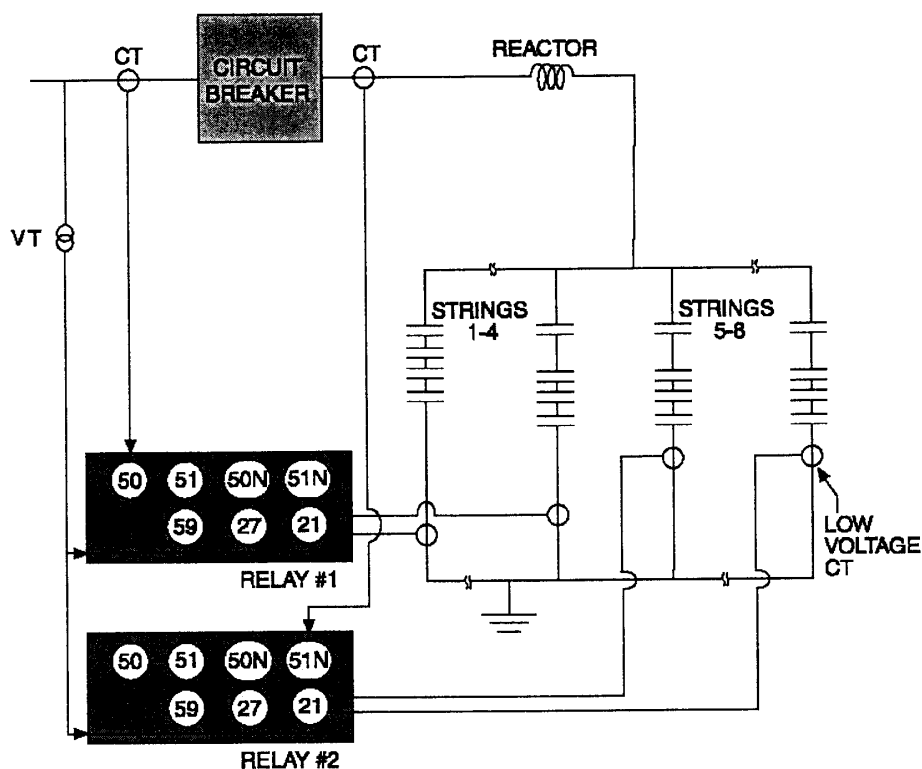
圖九：阻抗法的電容器組保護
