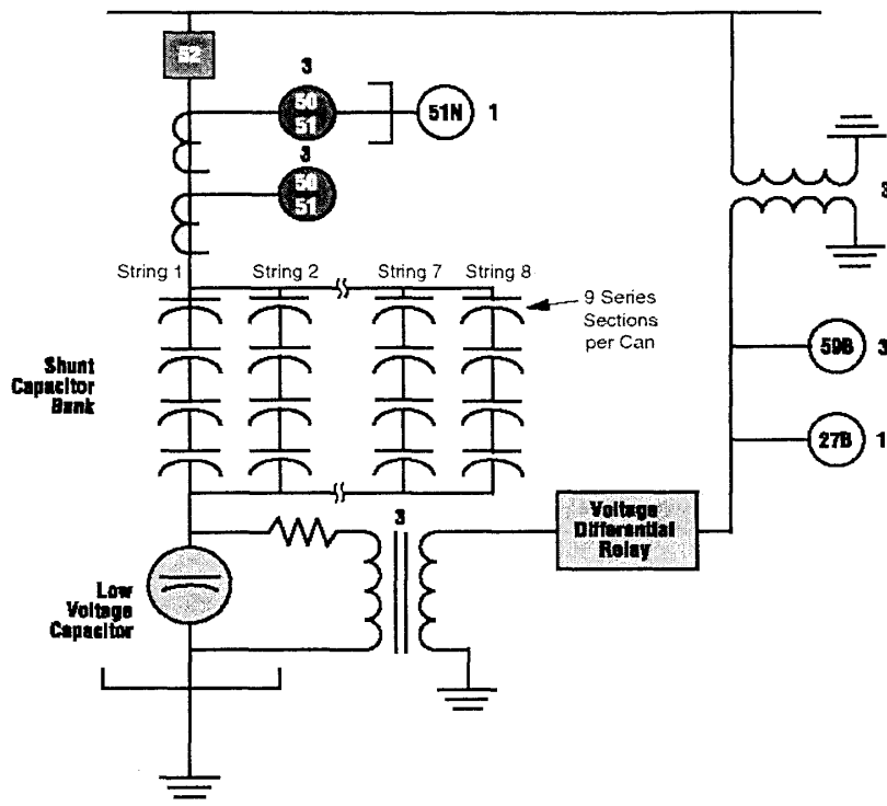
圖六：典型的電壓比較電容器組保護方式
