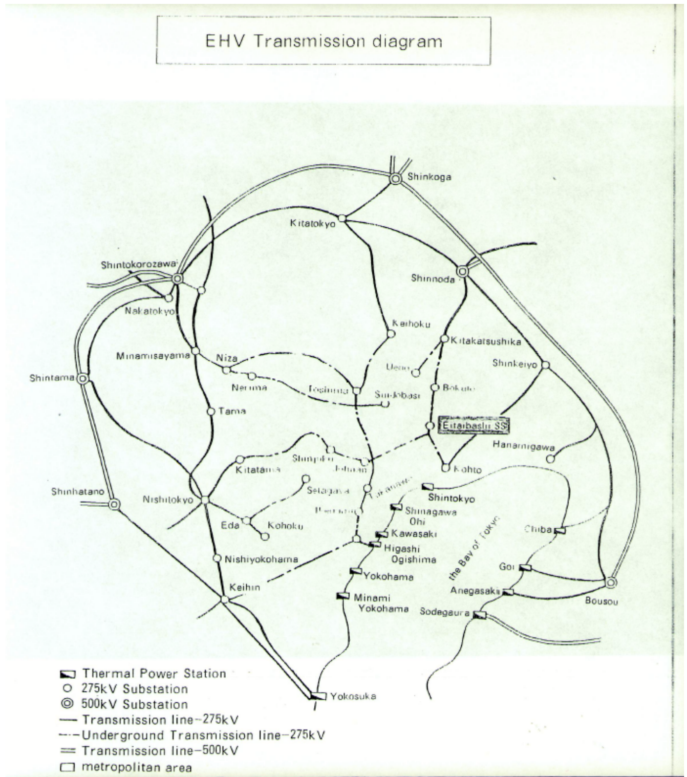
圖一.大東京都會區 275KV 輸電系統圖
