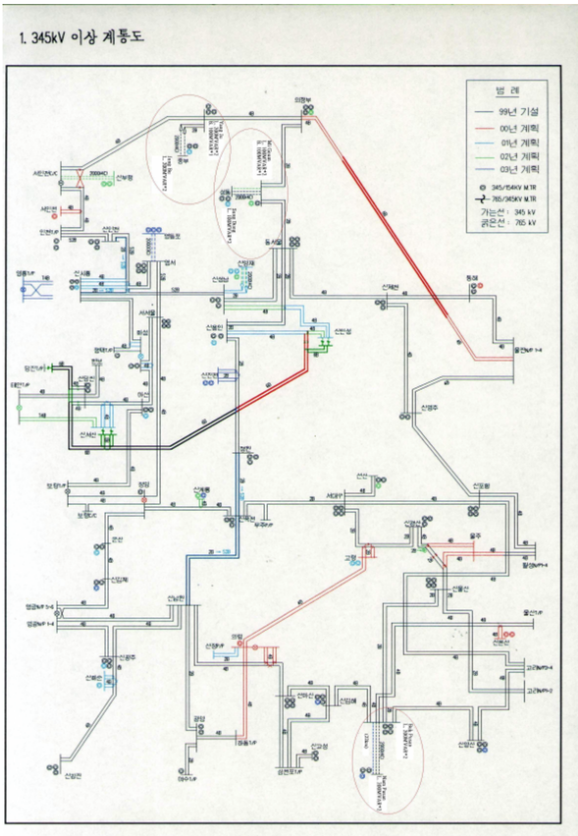
圖三.韓電 345KV 輸電系統圖
