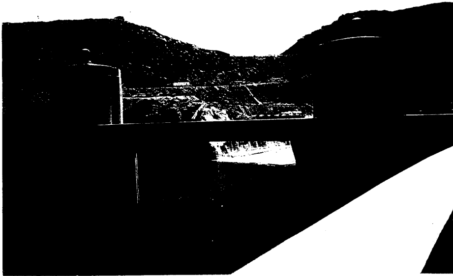
Hoover Dam 塔式取水口
