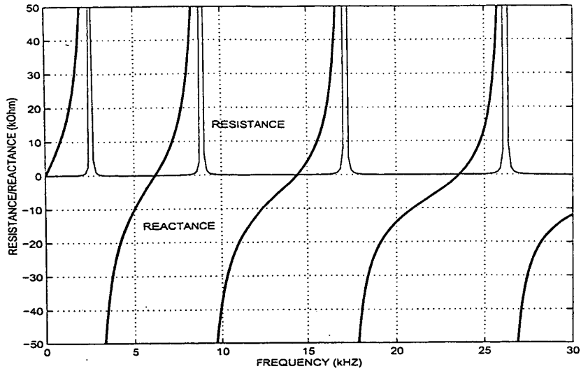
圖 4.5.1 線圈/繞組的阻抗與頻率關係
