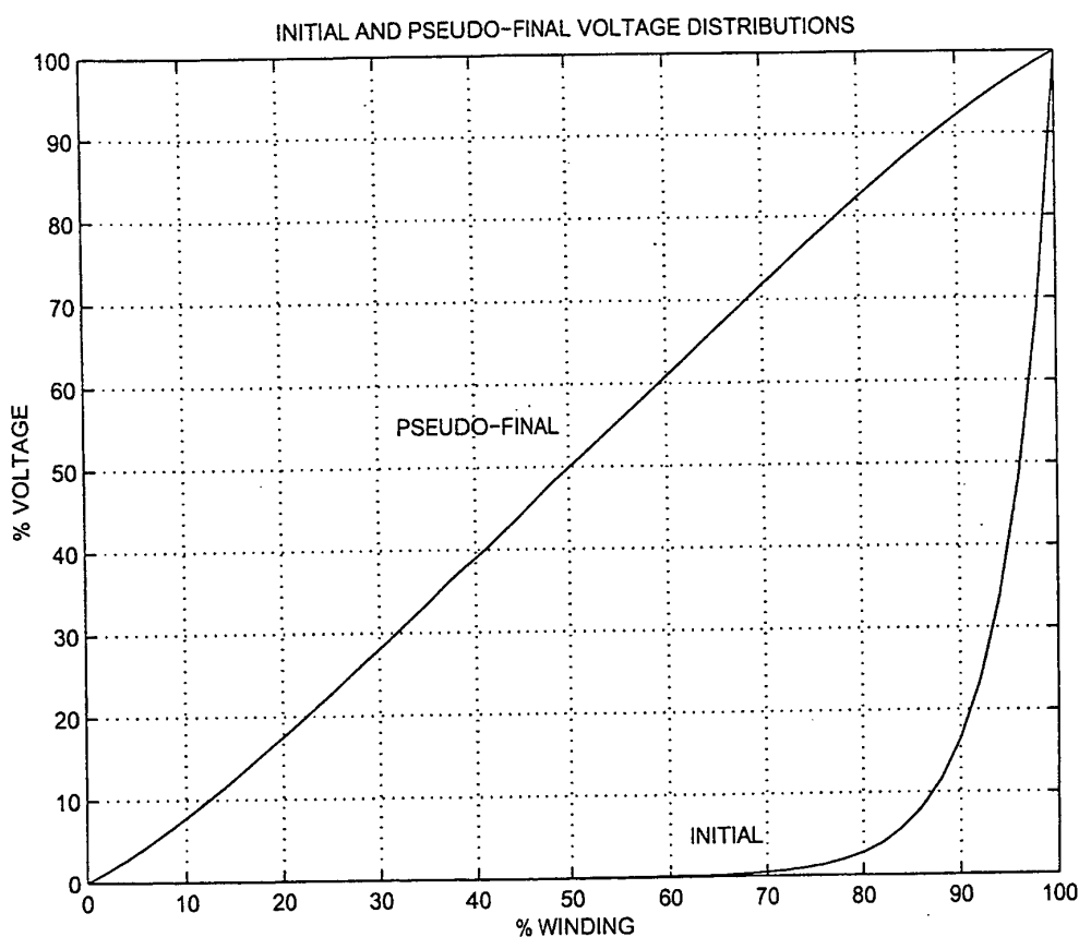
圖 4.4.1 線圈/繞組之時域暫態反應 (INITIAL：初始電壓/電流分佈期、PSEUDO-FINAL：電壓/電流週期震盪期)
