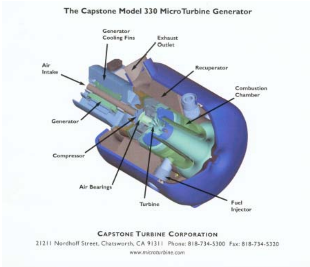
附圖二、微型氣渦輪發電機(Microturbine Generator)
