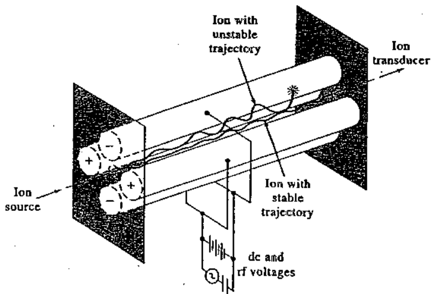
圖 8、傳統四極式質量分析器
