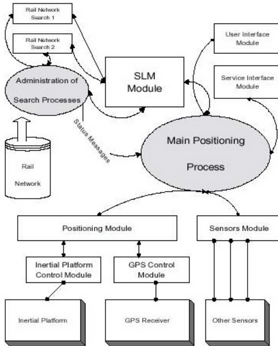
圖 16 SATURN light 的程序
