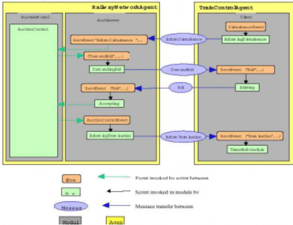
圖 23 各代理間的資訊流動
