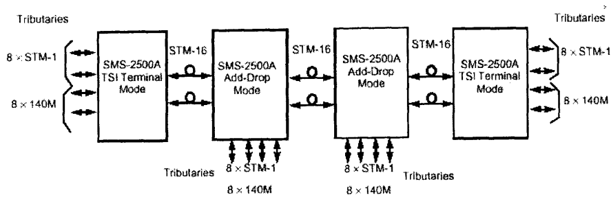
圖八 Linear ADM 系統示意圖
