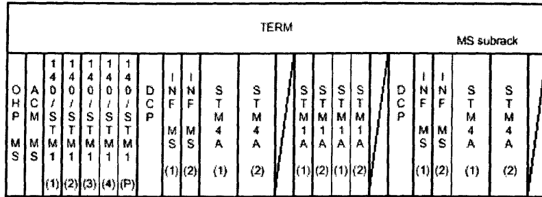
圖二 MS 機框配置圖
