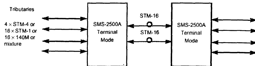
圖七 (a) Point to Point 系統示意圖
