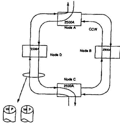
圖十 (a) 2F-BLSR~Normal
