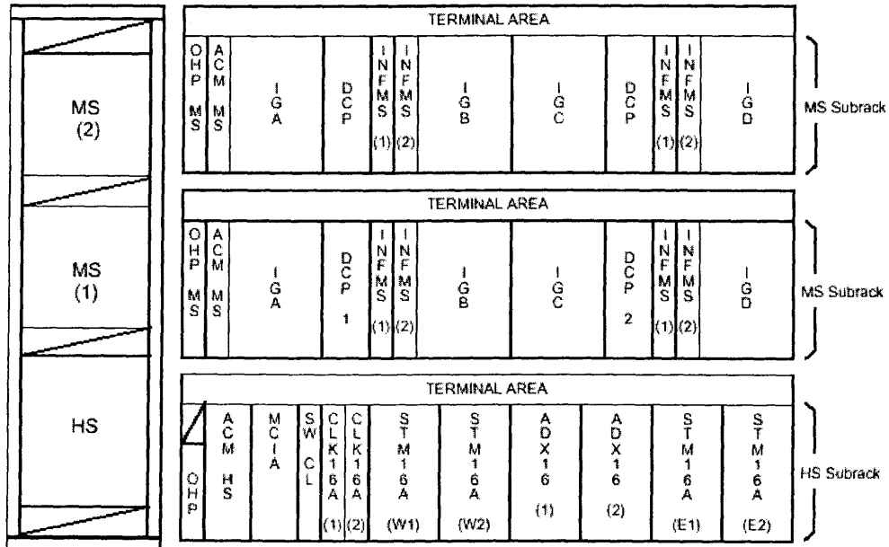
圖一 SMS-2500A 機架配置圖
