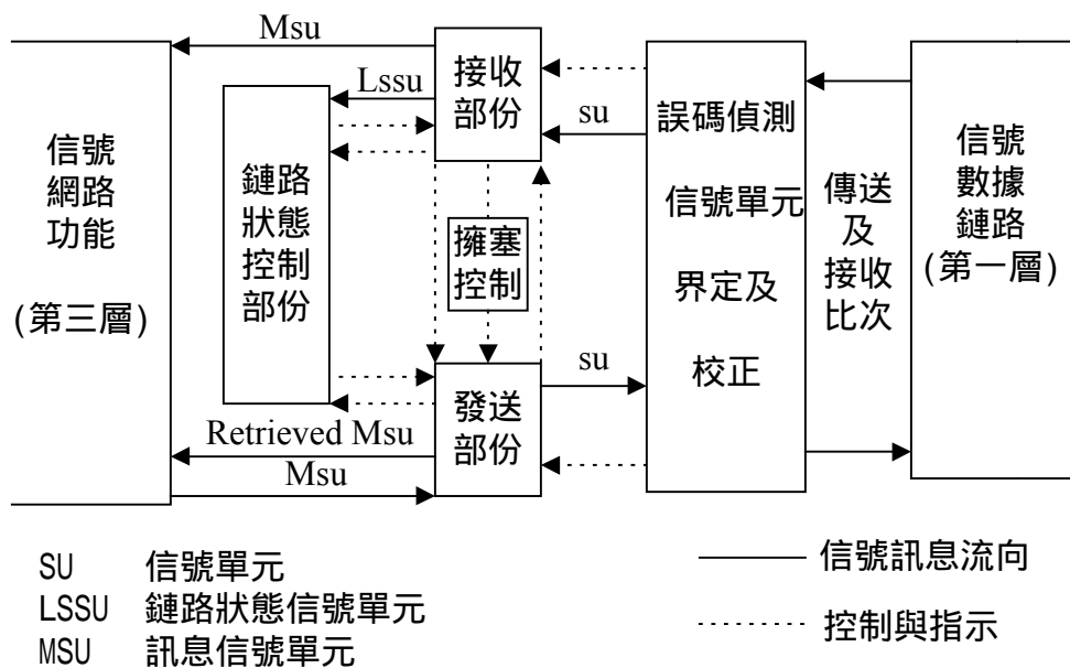
信號鏈路功能方塊圖
