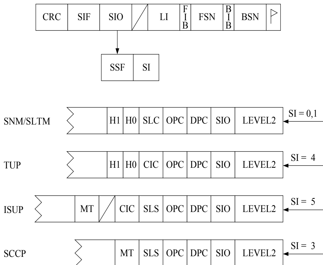
信號網路訊息格式圖
