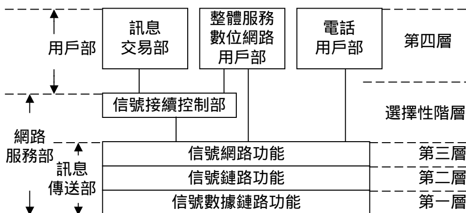
SS7 信號系統架構
