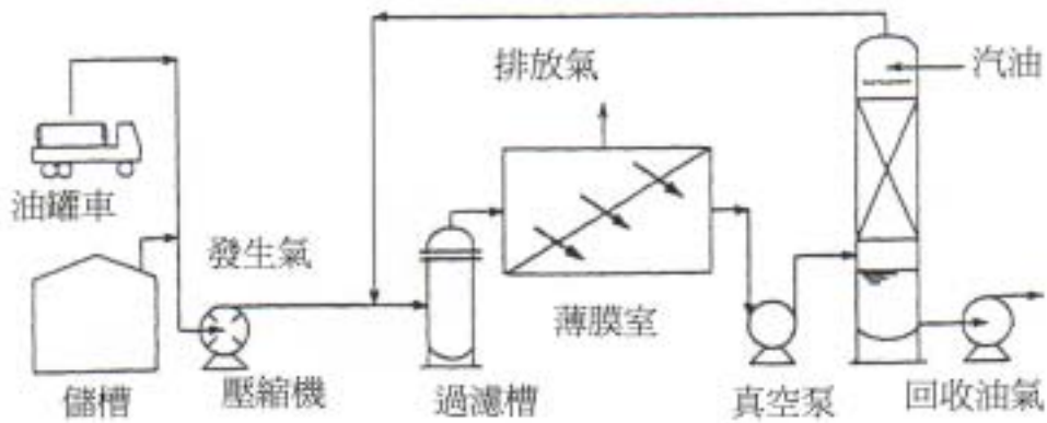
圖九、薄膜分離法
