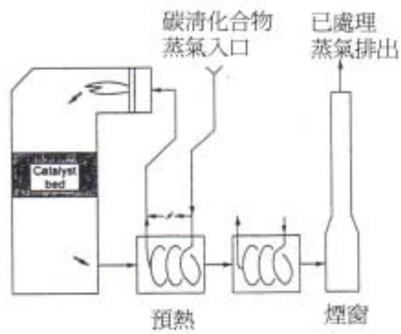
圖十一、燃燒法
