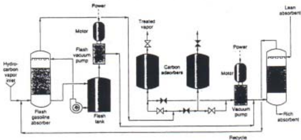
圖十二、吸收 + 吸著 ( 活性碳 ) + 吸收
