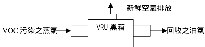
圖五、VRU 系統
