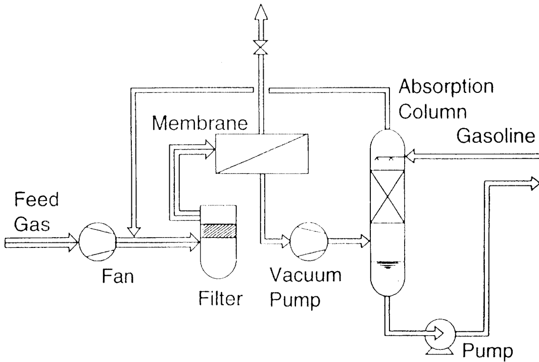
圖四、吸收—薄膜—吸附式
