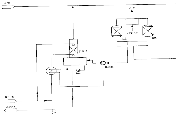
圖二、活性炭吸附式
