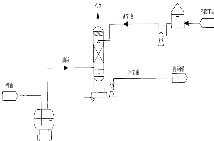
圖一、重油吸收式
