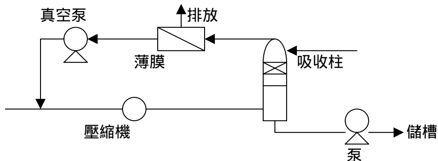
圖六、油氣回收系統
