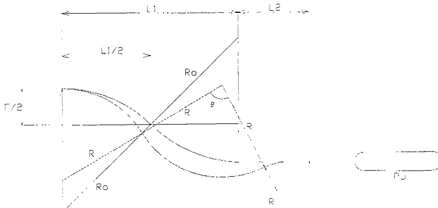
圖 2、電纜之 OFF-SET 圖
