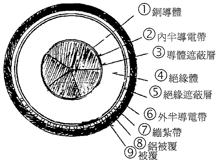
圖1、345KV 交連 PE 電纜剖面圖
