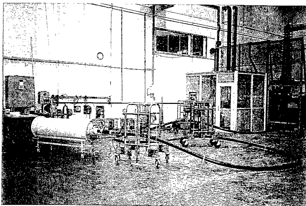
附圖九：接頭測試之情形
