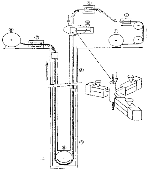
附圖六：CCV(懸垂鏈式交連硫化)製造設備概示
