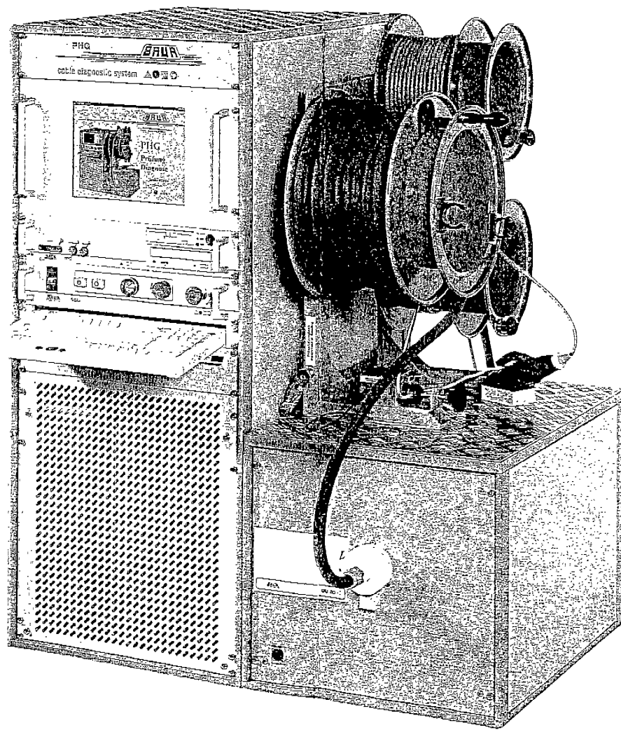
附圖三：VLF 測試設備
