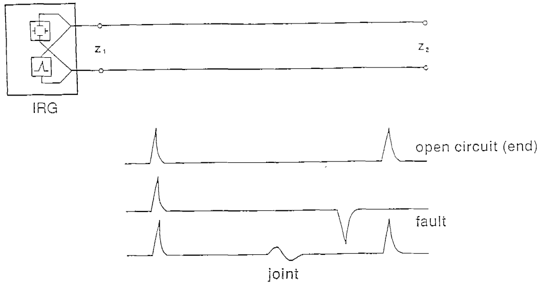
附圖一：突波反射法之接線方式及反射波形
