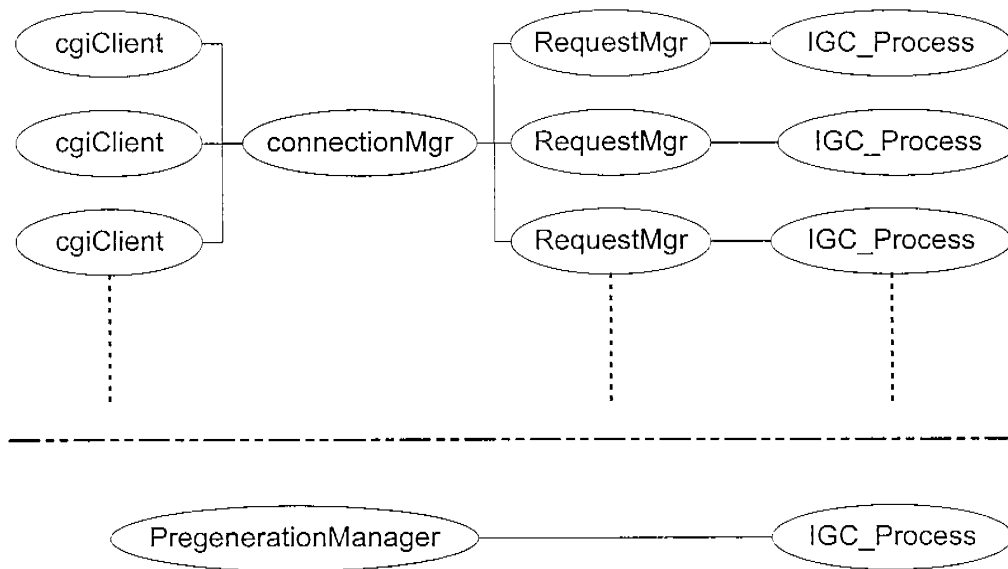
圖二 FX-Net伺服器端軟體架構
