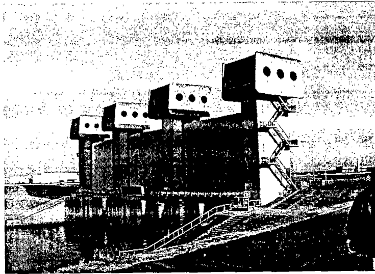
圖四、荒川與隅田川匯流新設閘門
