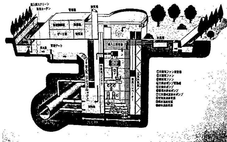
横斷示意圖 圖三、神田川環七地下河川取水設施
