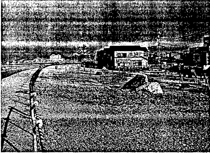
圖十三、淀川枚方市高規格堤防
