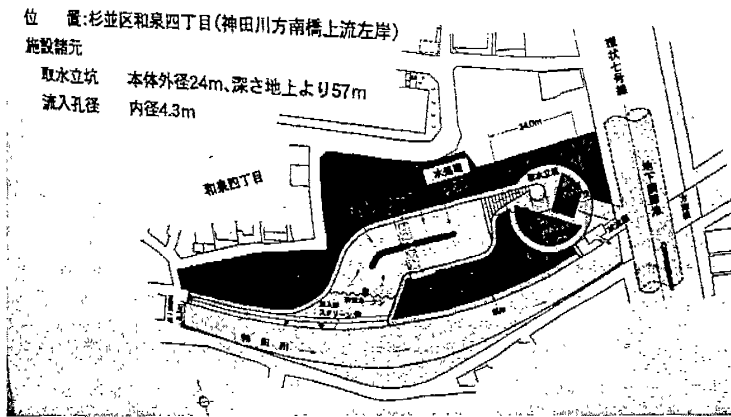
面佈置圖 圖二、神田川環七地下河川取水設平
