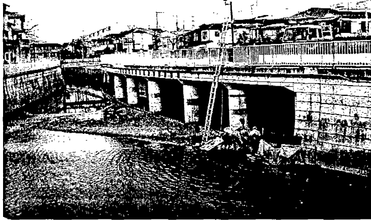
口 圖一、神田川環七地下河川越流堰入
