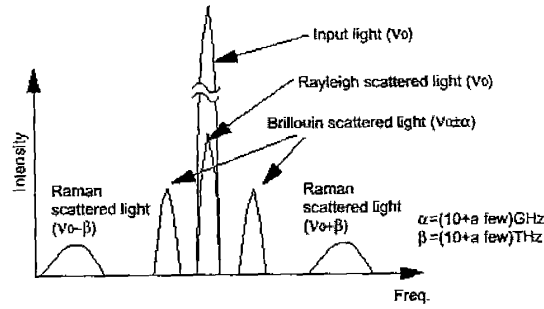
圖4.1.2 典型散射光譜
