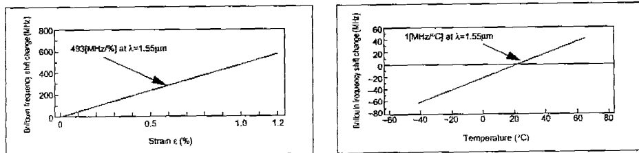
圖4.1.3 布里努恩頻率移動量與應變及溫度之關係
