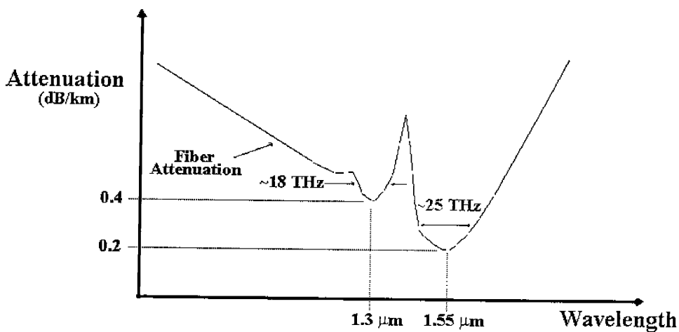
圖 3.1.1 光波長損失及頻寬圖
