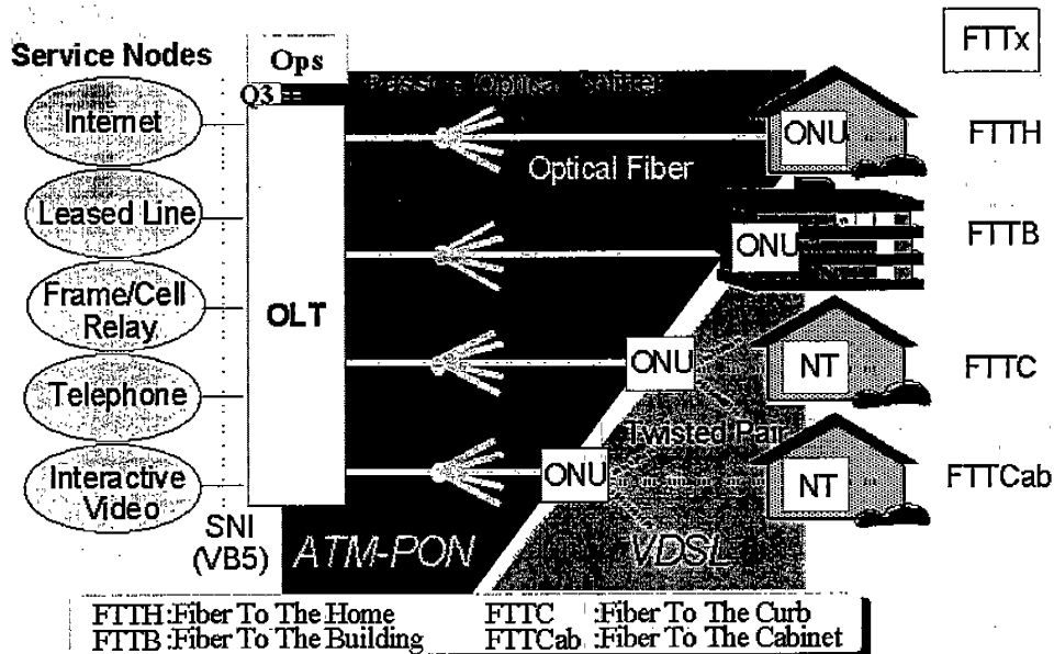
圖2.3.1 FTTx用戶迴路ATM-PON存取系統
