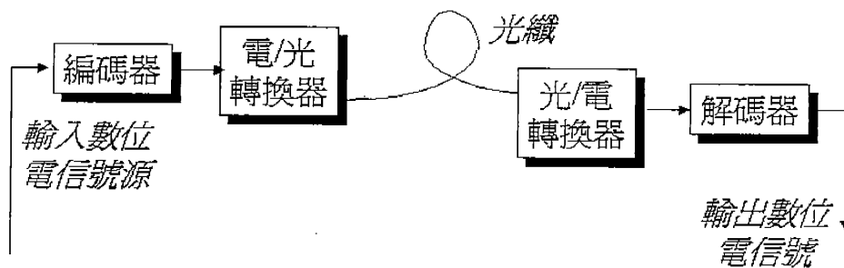
圖 2.1.2 典型光纖通訊系統方塊圖
