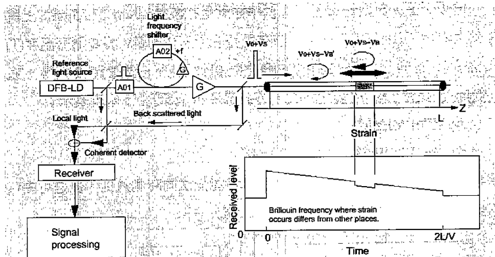
圖4.1.4 AQ8602 基本組態和信號波形
