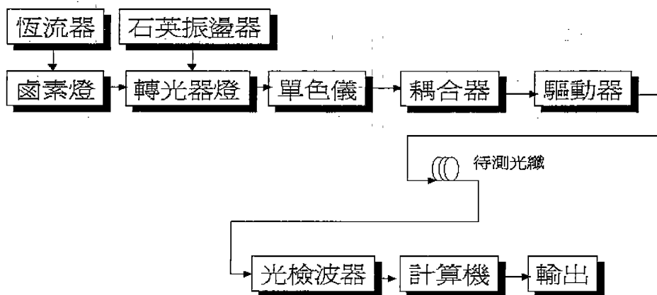
圖3.2.4 光纖損耗譜檢測系統
