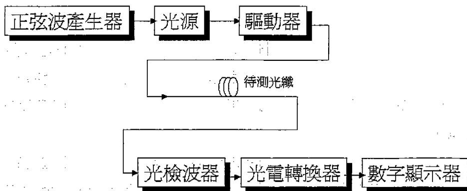
圖3.2.3 插入法檢測光纖損耗系統方塊圖
