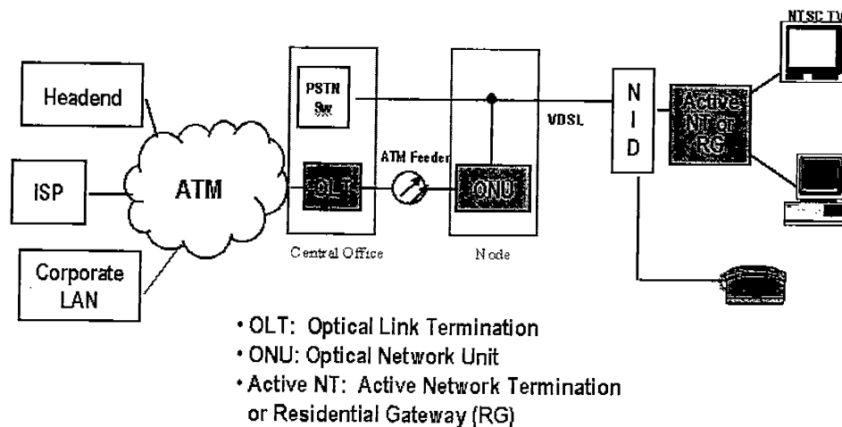
圖2.3.2 FTTC+VDSL方案示意圖
