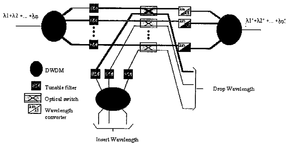
圖 2.1.3 未來之光交換網路
