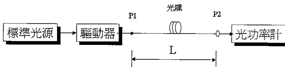
圖3.2.2 剪斷法檢測光纖損耗系統方塊圖
