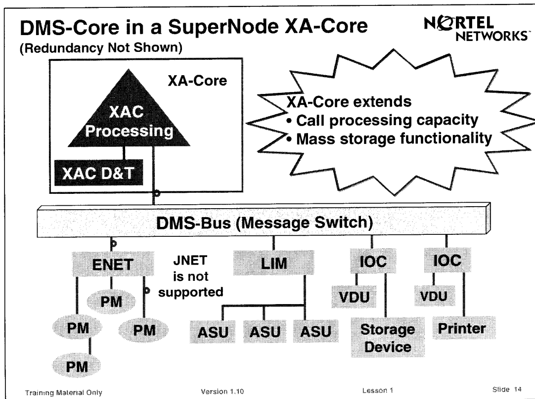
圖 1.1 XA-Core 交換機架構
