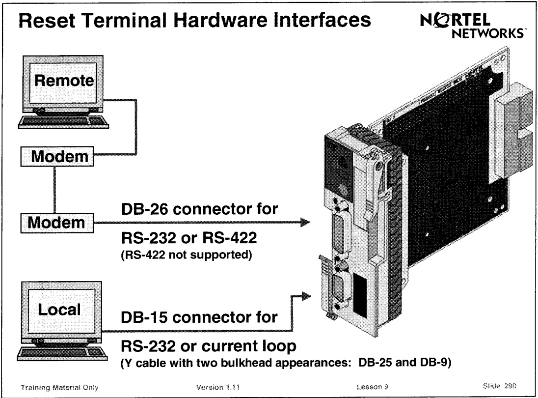
圖 9-11 Reset terminal 硬體連接圖
