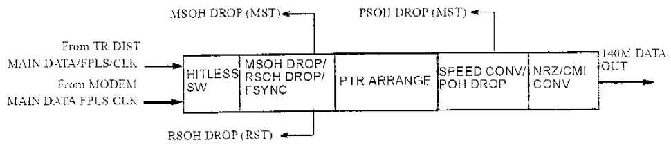
圖 3-26 140M 介面模組之接收端信號處理流程
