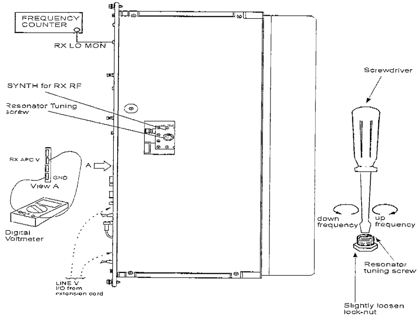
圖 3-32 備用單體之接收頻率調整
