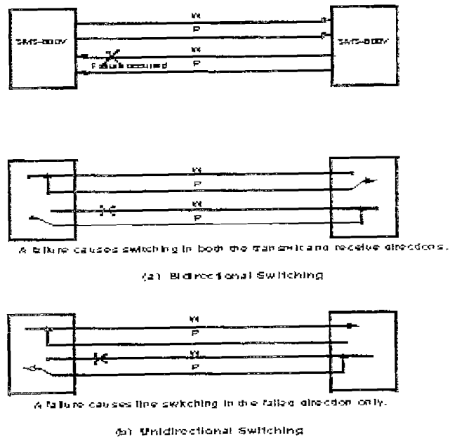
圖5.4.10 線路保護方式
