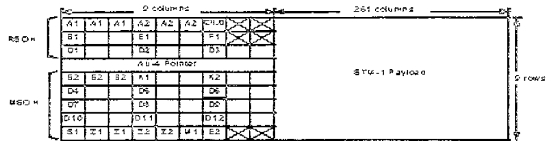
圖5.2.2 SMS-600V其碼框的標頭位元組
