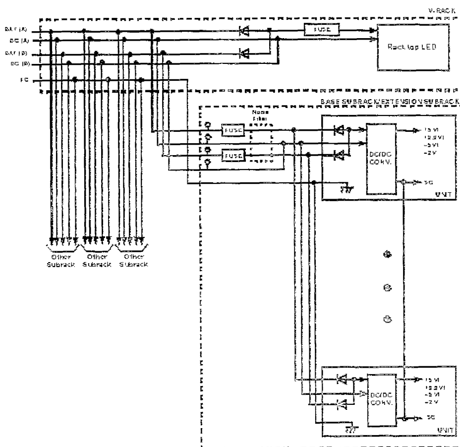
圖5.8.1 SMS-600V電力分配方式
