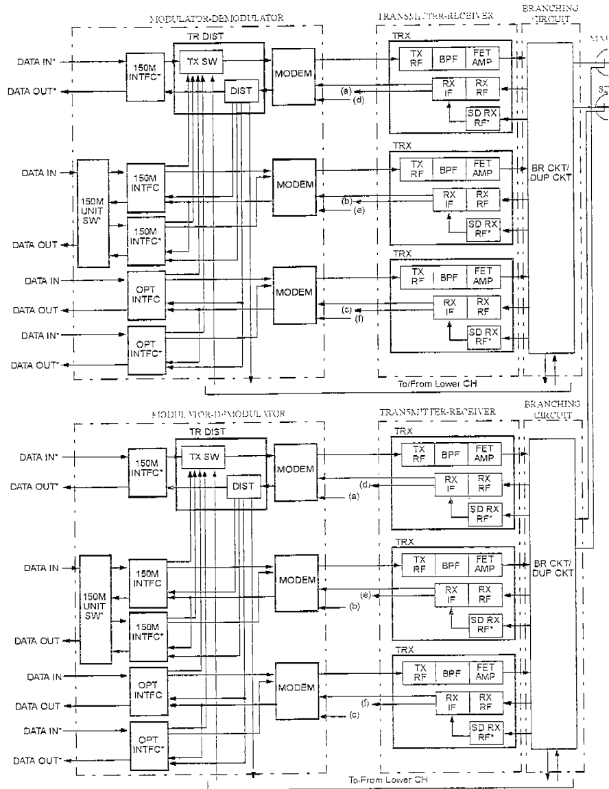
圖 3-10 具有 140M,150M 電介面及 OPT 光介面之終端站系統方塊圖 (採 2+1 XPIC 系統架構)
