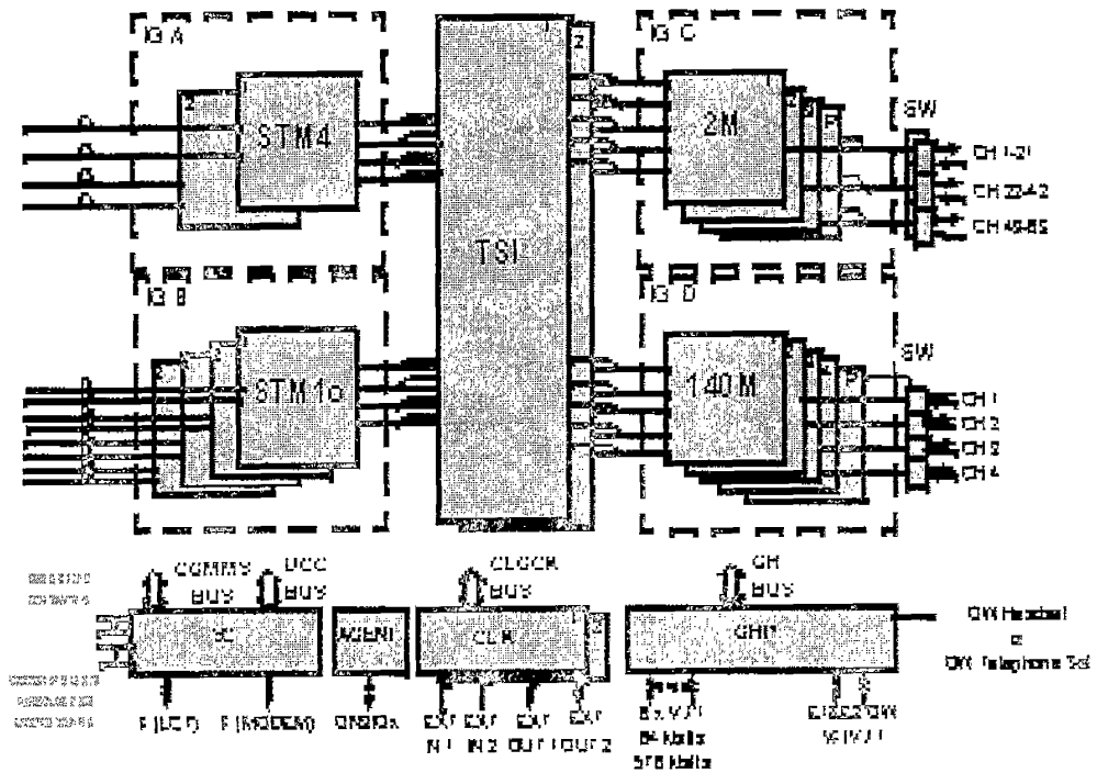
圖5.5.1 SMS-600V之功能方塊圖
