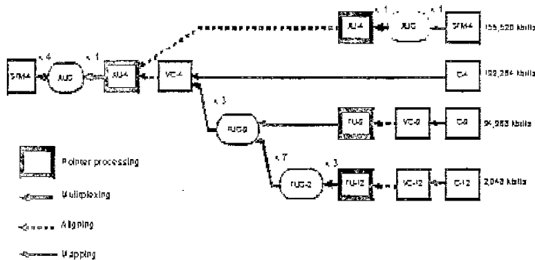
圖5.2.1 SMS-600V訊號流與映射架構
