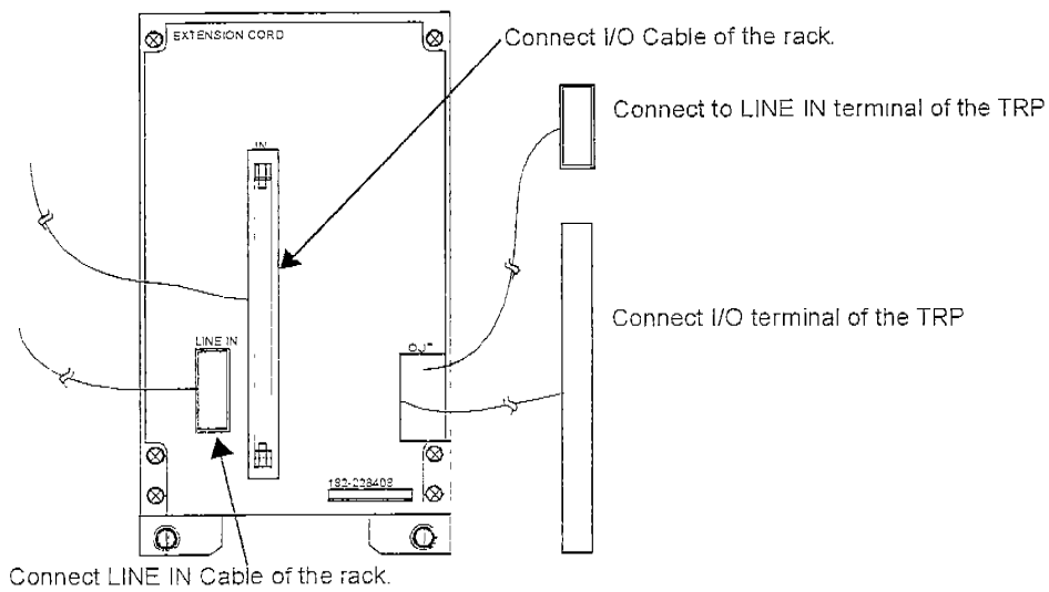
圖 3-29 TRP 延伸線
