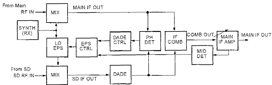
圖 3-22 接收端中頻信號轉換及組合
