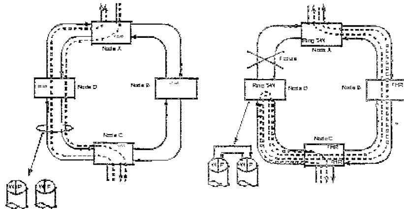
圖5.4.7 2-FIBER BLSR(2F MS-SP)
