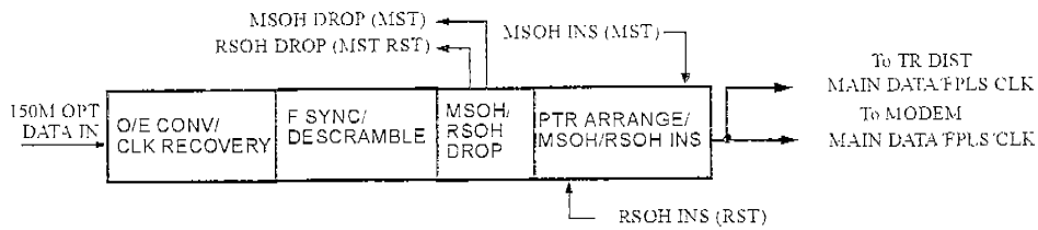
圖 3-17 光介面模組之發送端信號處理流程
