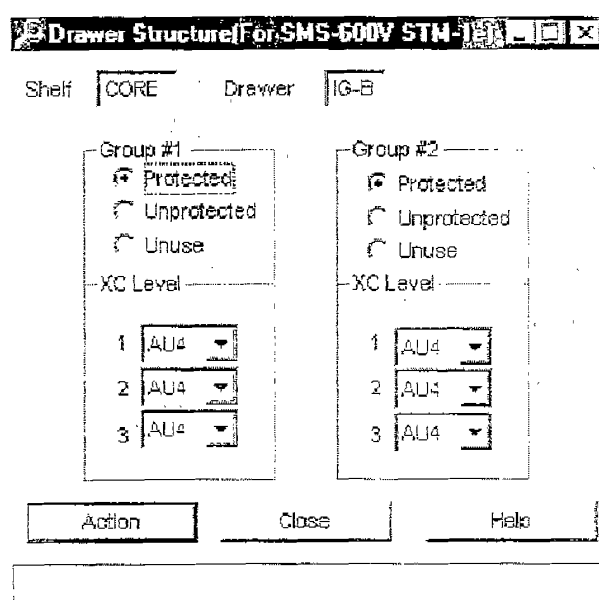
SMS-600v, STM-1e ADM。圖 4.37
