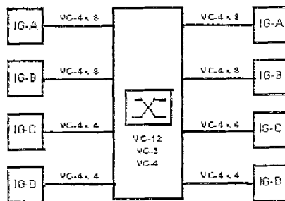
圖5.6.1 時槽交接单體功能方塊圖
