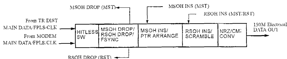
圖 3-24 150M 介面模組之接收端信號處理流程
