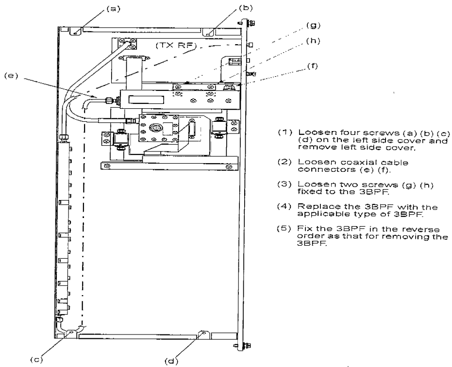
圖 3-31 更換 3BPF
