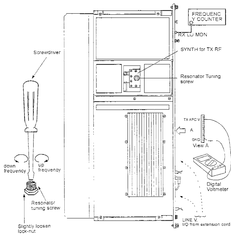
圖 3-30 備用單體之發射頻率調整
