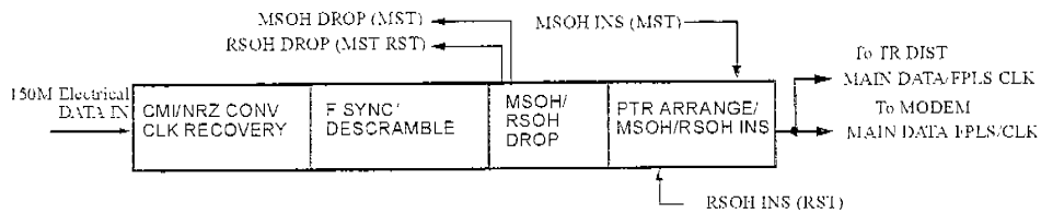
圖 3-16 150M 介面模組之發送端信號處理流程
