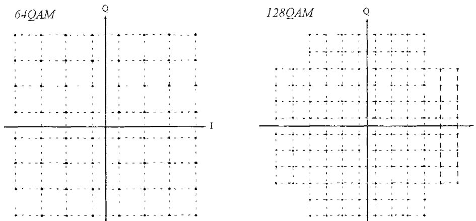
圖 3-20 64QAM/128QAM 星座圖
