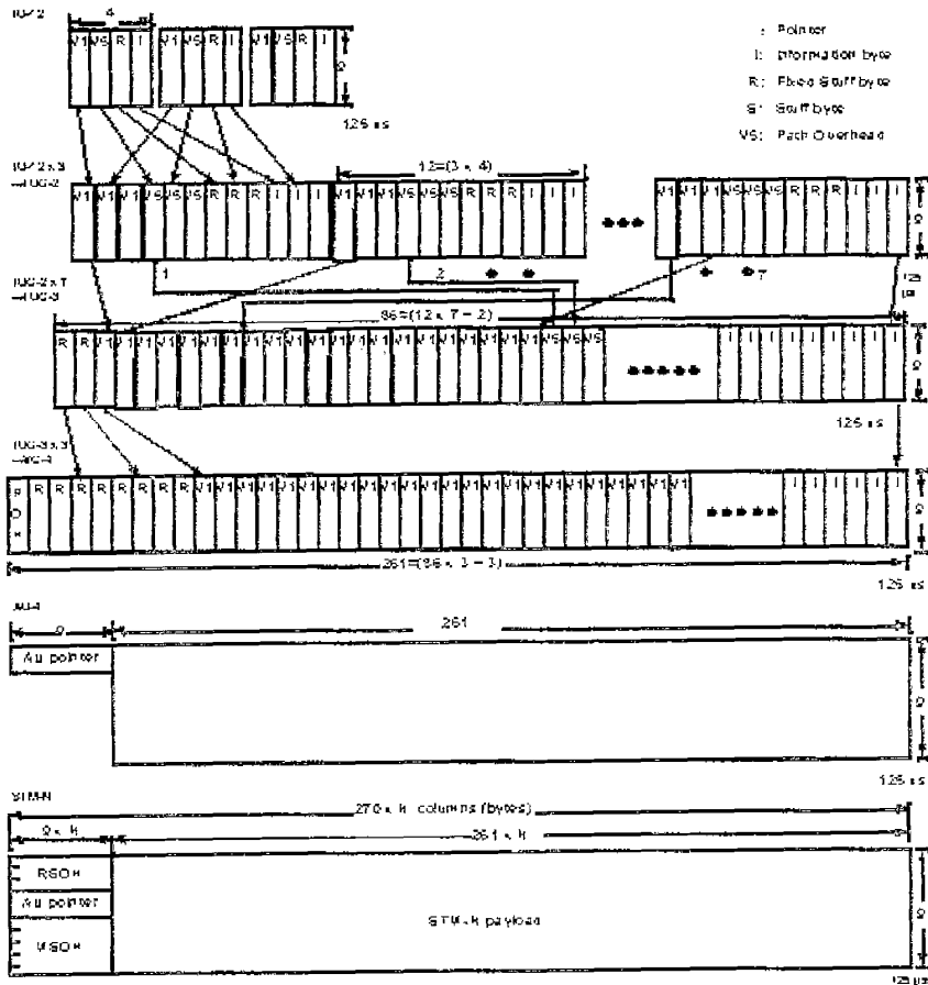
圖5.2.4 SMS-600V其碼框處理架構
