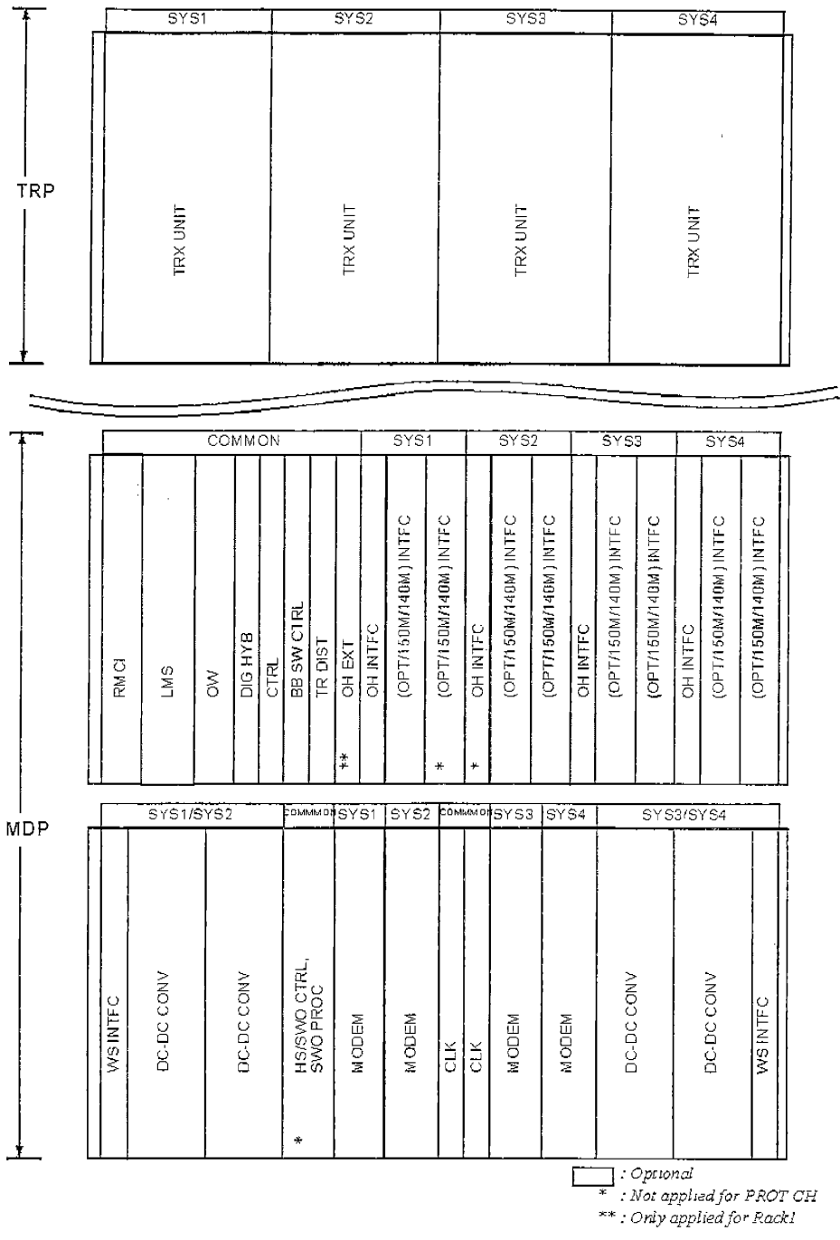
圖 3-5 3000S SDH 數位微波設備機架單體排列圖
