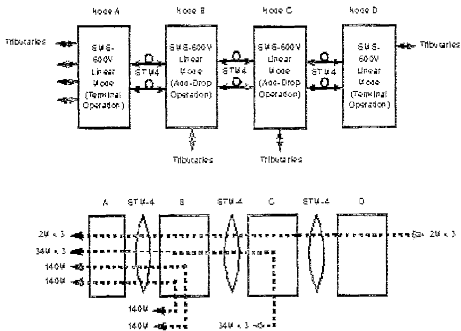
圖5.4.3 Center-to-Node System應用架構圖
