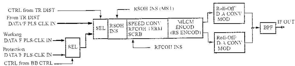
圖 3-19 調變解調器模組之發送端信號處理流程
