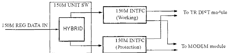
圖 3-14 利用 150M UNIT SW 模組進行數位信號分配
