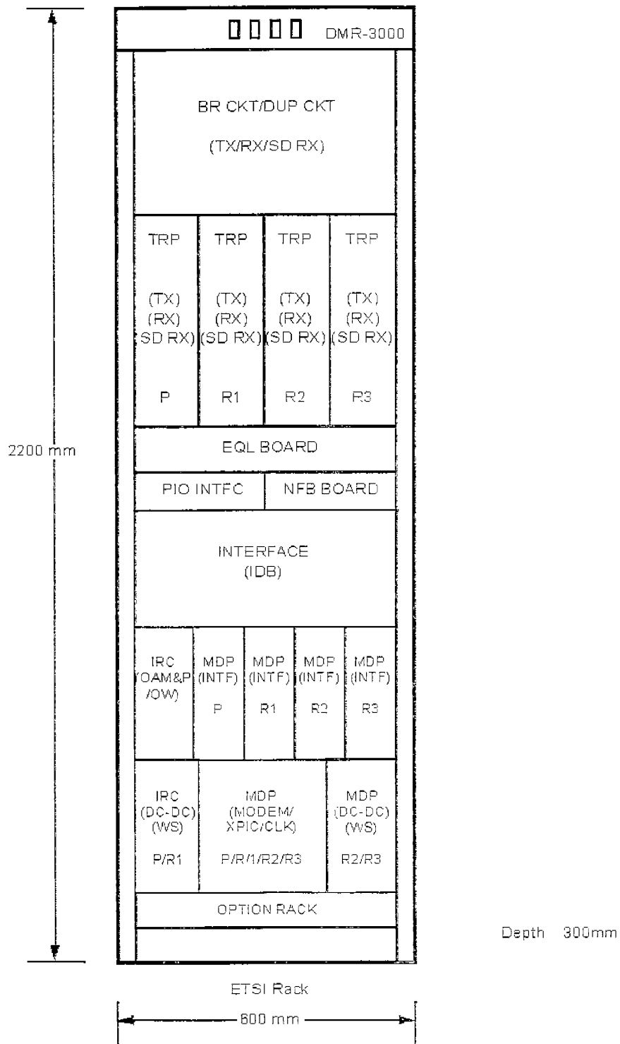
圖 3-4 3+1 系統之設備組態
