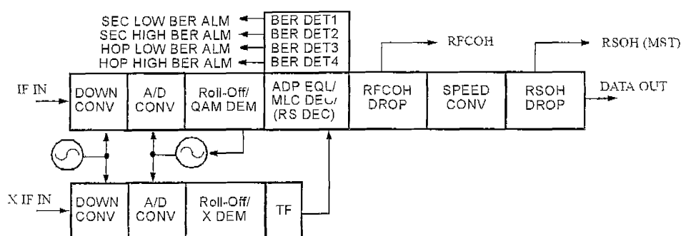
圖 3-23 調變解調器模組之接收端信號處理流程
