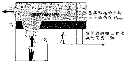
fig. 8 蓄煙可能容積
