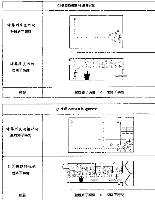
降時間較慢。 Fig.3 樓層避難安全檢証的過程
