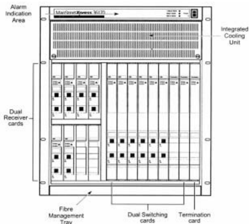
圖 3-5(a). Alcatel 7470 MSP 交換機架外觀圖
