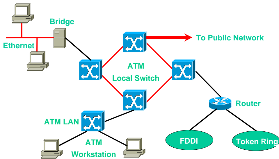
圖2.22 ATM骨幹的區域網路架構
