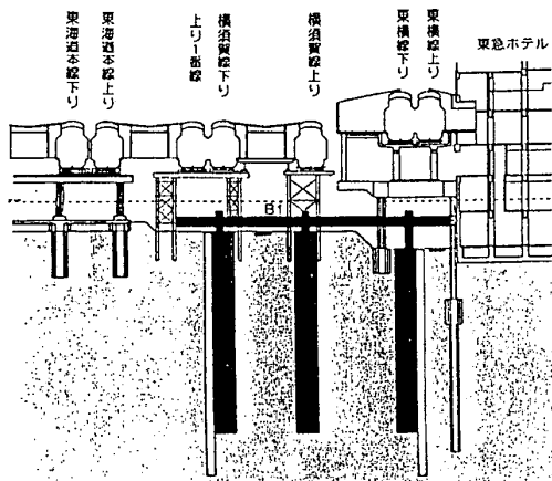
圖 5-3 横濱車站中央部份施工步驟示意圖
