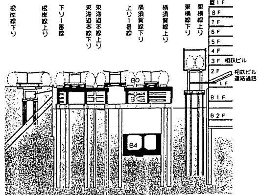
B4階<体構築工 B0軌道階<体構築工
