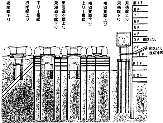
軌道仮受工 一次掘削
