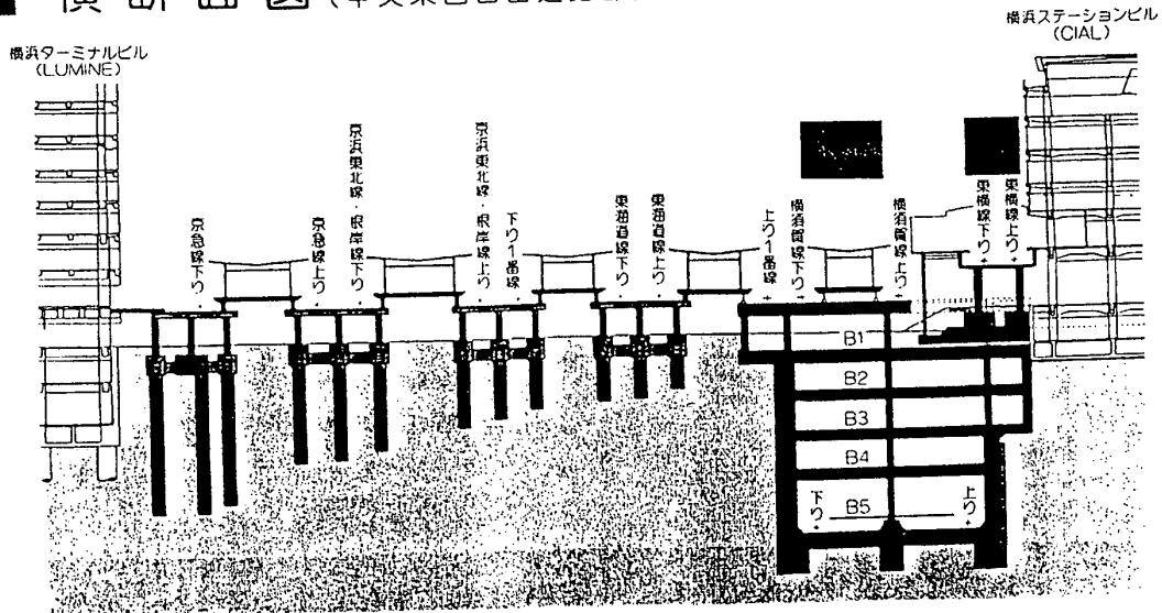
圖 5-1 橫濱車站之平面、縱断面與橫断面圖
