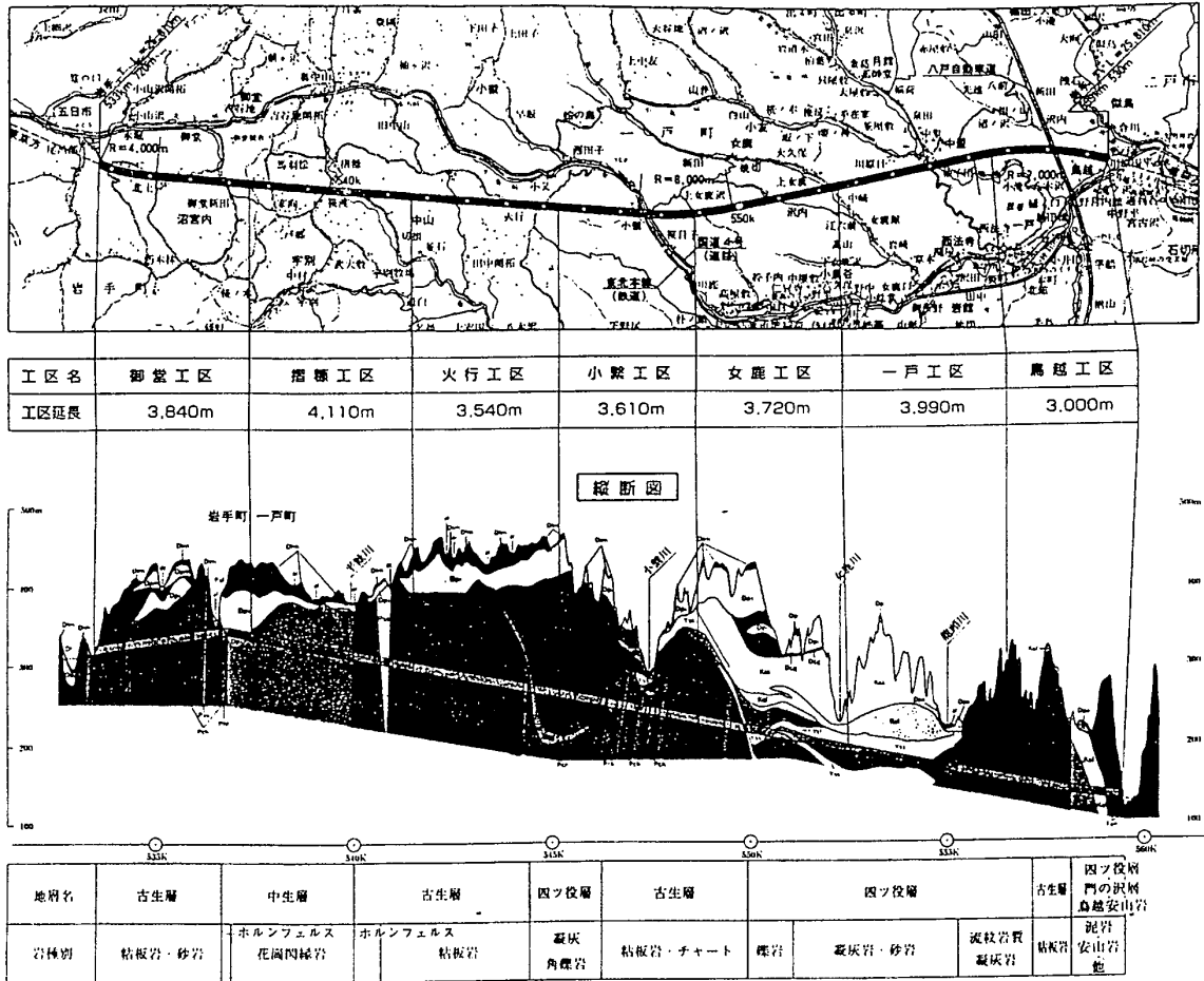
圖 4-1 岩手~一戸隧道地質之平縱斷面與工區名稱位置圖
