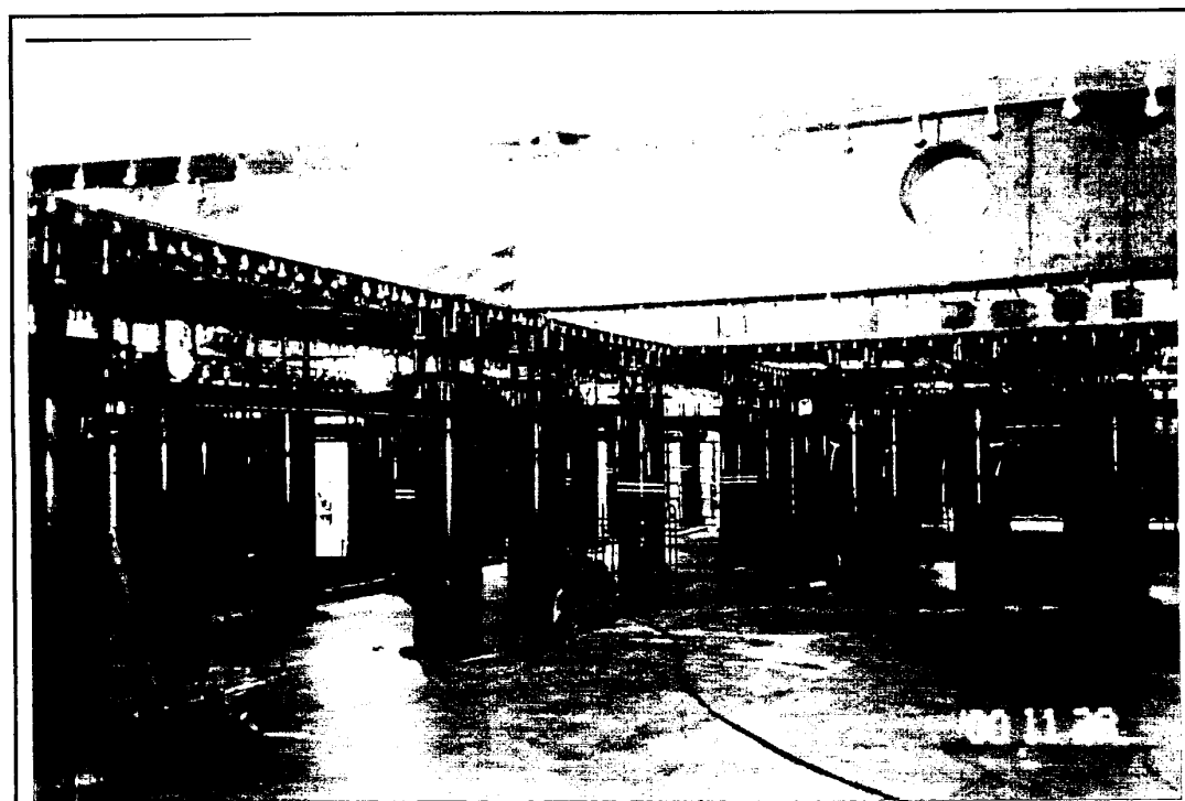
鋼管樁支撐與澆置完成之基礎版
