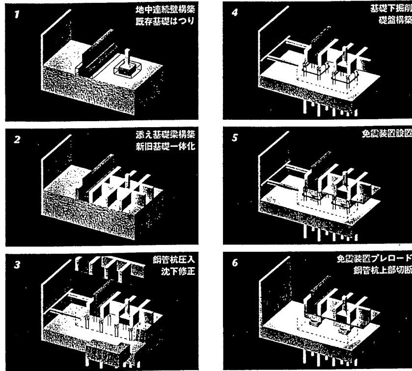
圖 1-2 施工步驟示意圖
