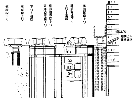
東急高架橋撤去 II期工事施工
