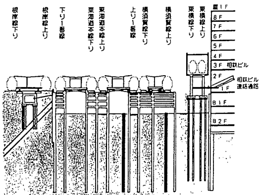
地下連続壁施工
