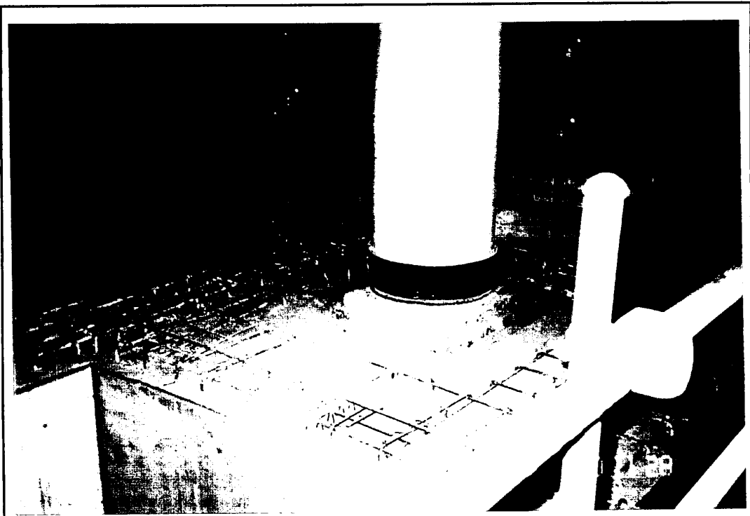
既有基礎與新設基礎之結合
