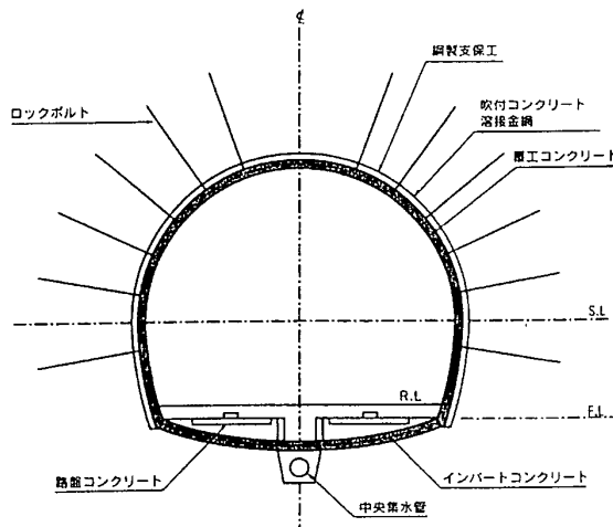
圖 4-3 岩手~一戶隧道標準斷面圖
