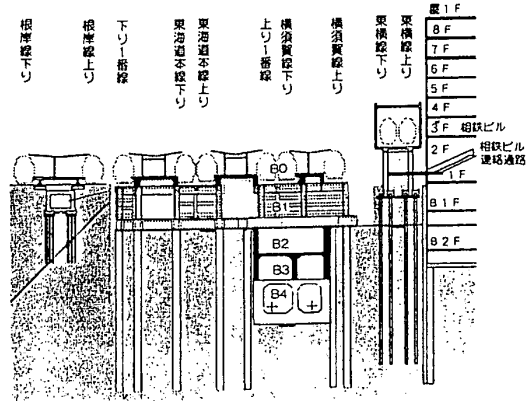
B3~B2階<体構築工
