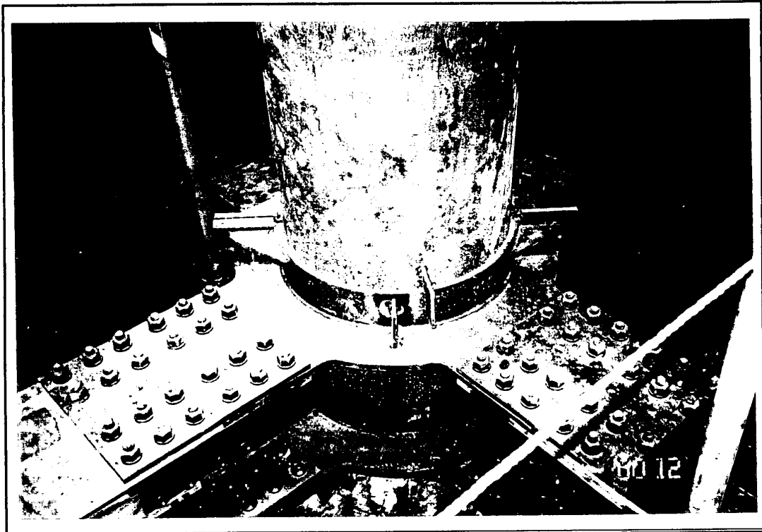
鋼管樁支撐處之接合
