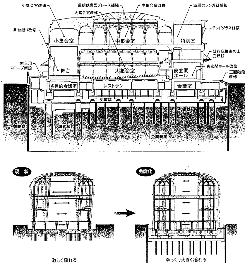
圖 1-1 減震設施之功能示意圖
