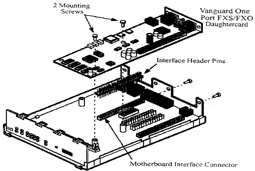
圖 9 語音卡的裝置
