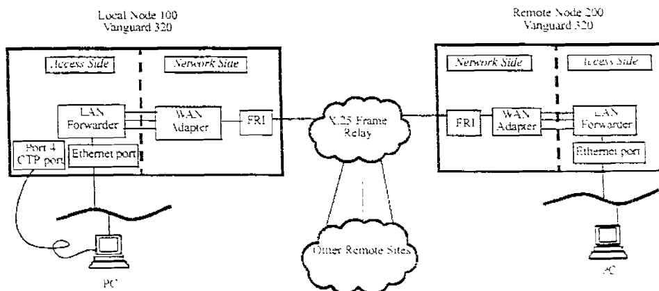
圖 13-1 網路範例 Figure 3-1. Sample Network
