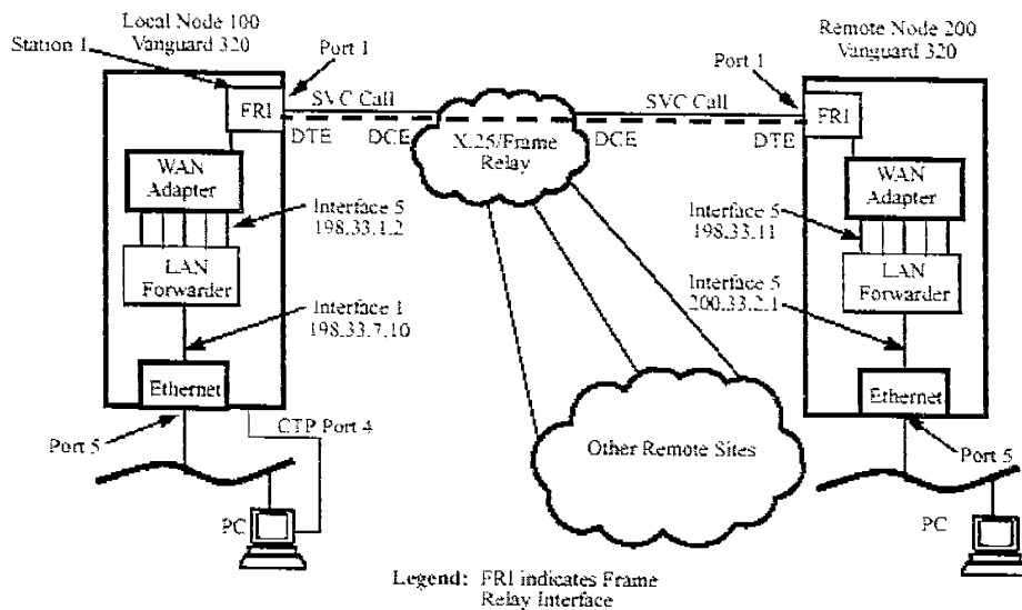
圖 15-1 LAN 介面設定範例
