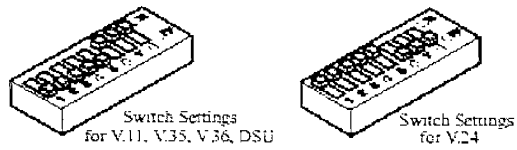
圖 4-2 設定 DIM 的指撥開關
