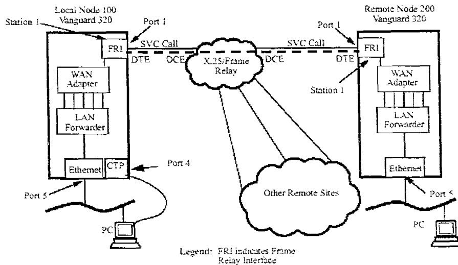
圖 12-4 WAN 介面設定範例
