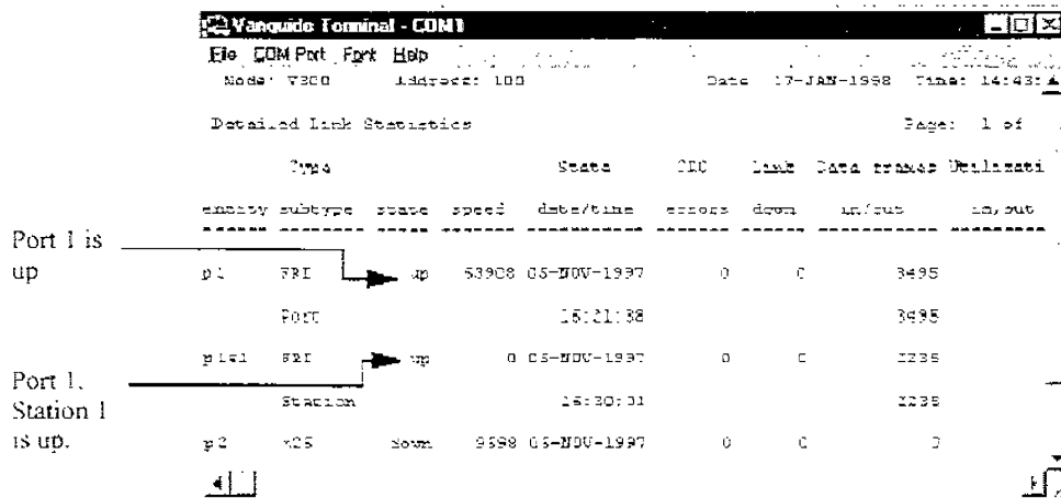
圖 14 詳細的連結狀態統計畫面
