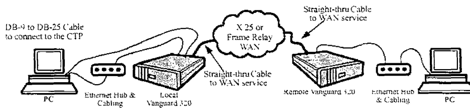
圖 12-3 Vanguard 320 網路接線範例
