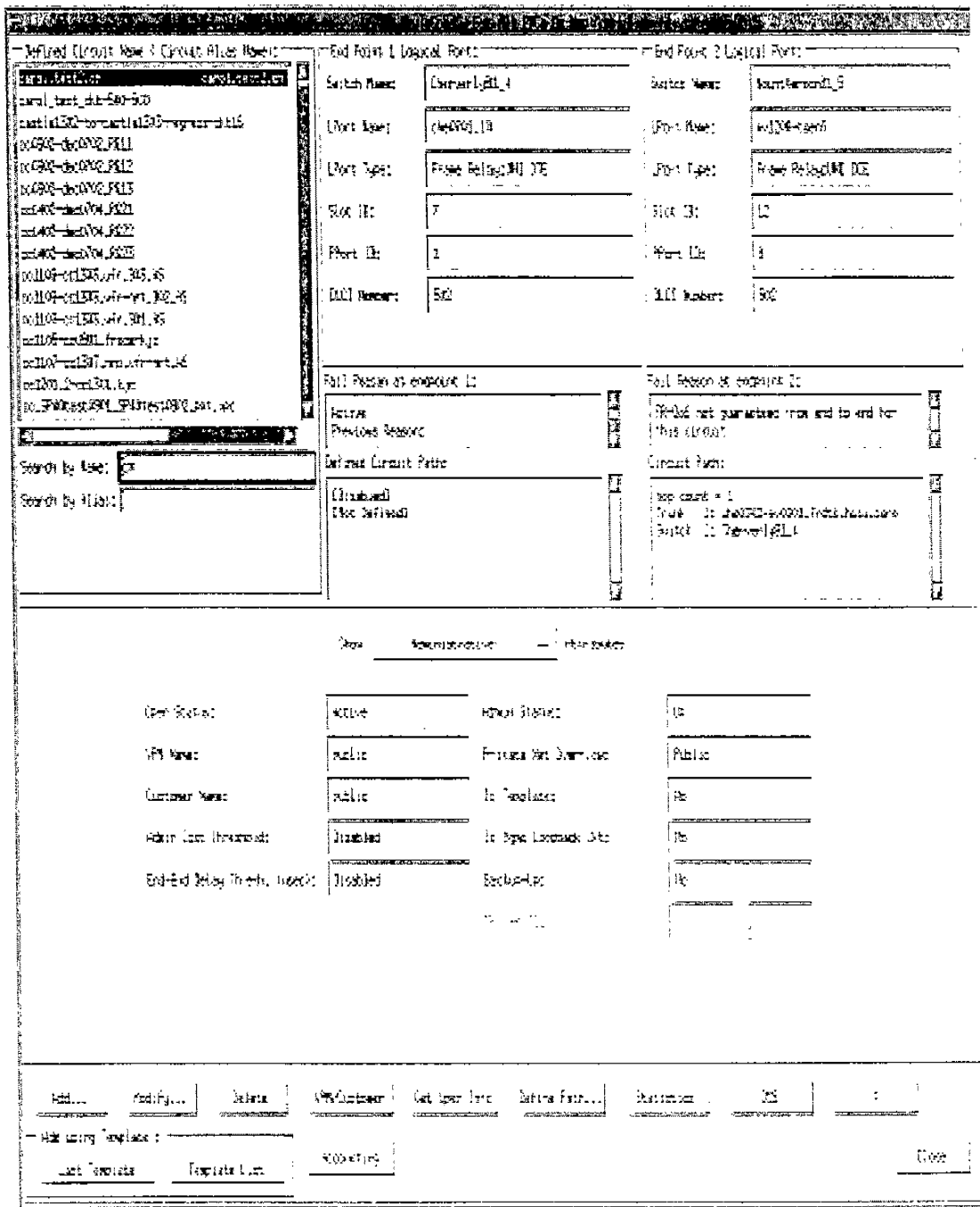
圖 II-4、「Set All PVCs on Map」對話框
