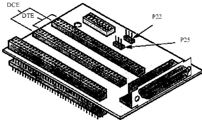
圖 4-1 DIM Site Daughtercard
