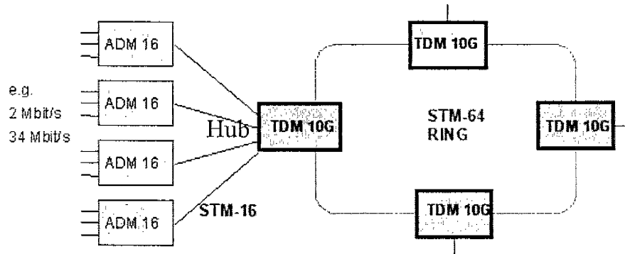
圖六 Ring & Hubbing
