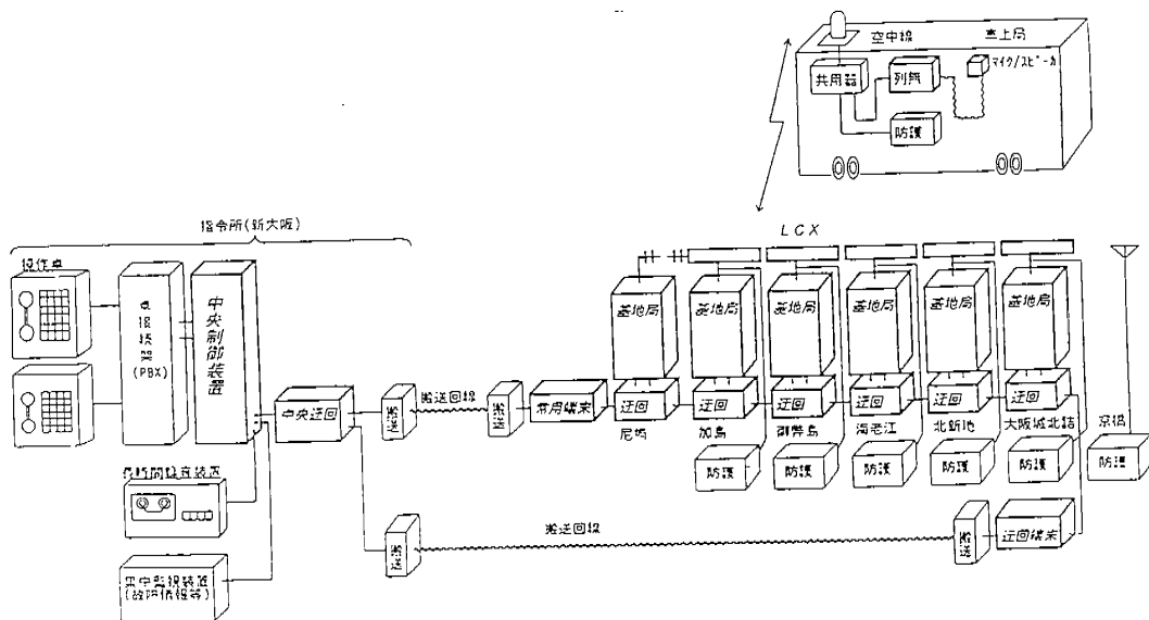
圖一、列車調度無線電話系統架構示意圖
