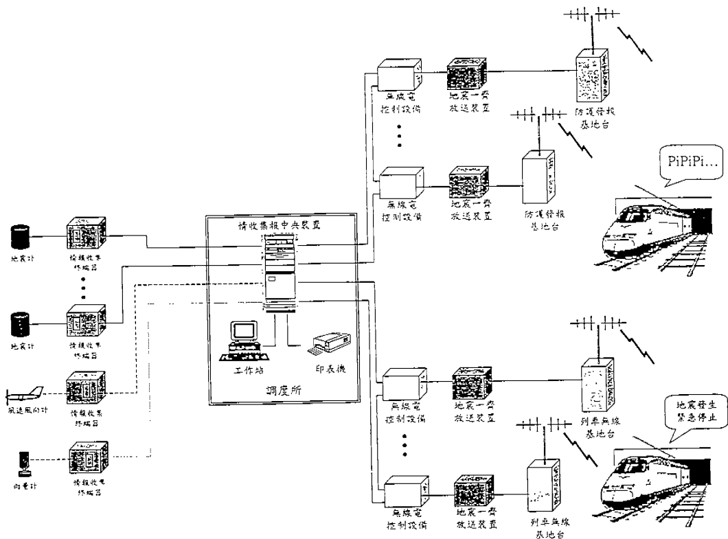
圖二、地震情報早期傳送架構示意圖
