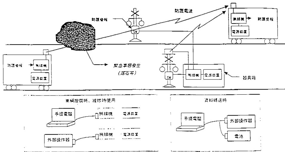
防護無線電設備之構成
