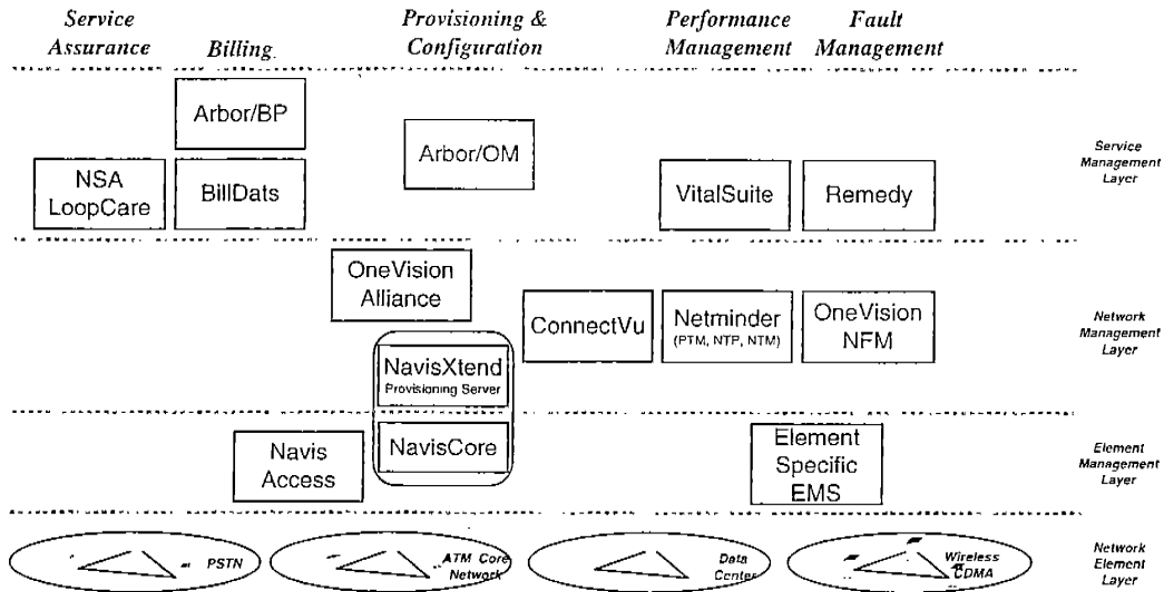
圖 3.1 整合網路及服務管理系統
