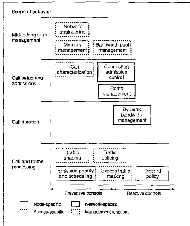
圖 1.3.2 訊務管理
