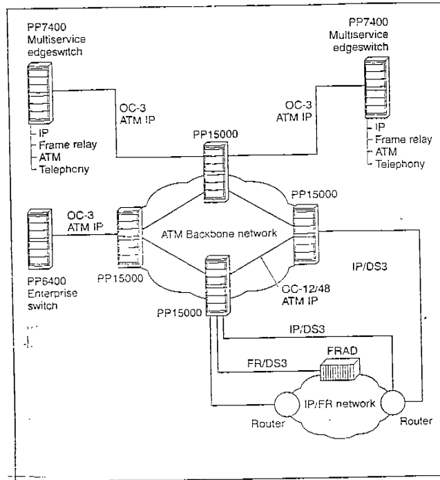
圖 1.1 ATM 網路示意圖
