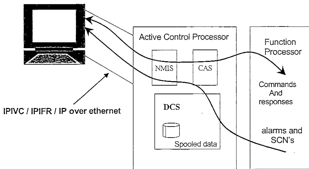
圖 2.2.3-1 Passport 網管連接方式
