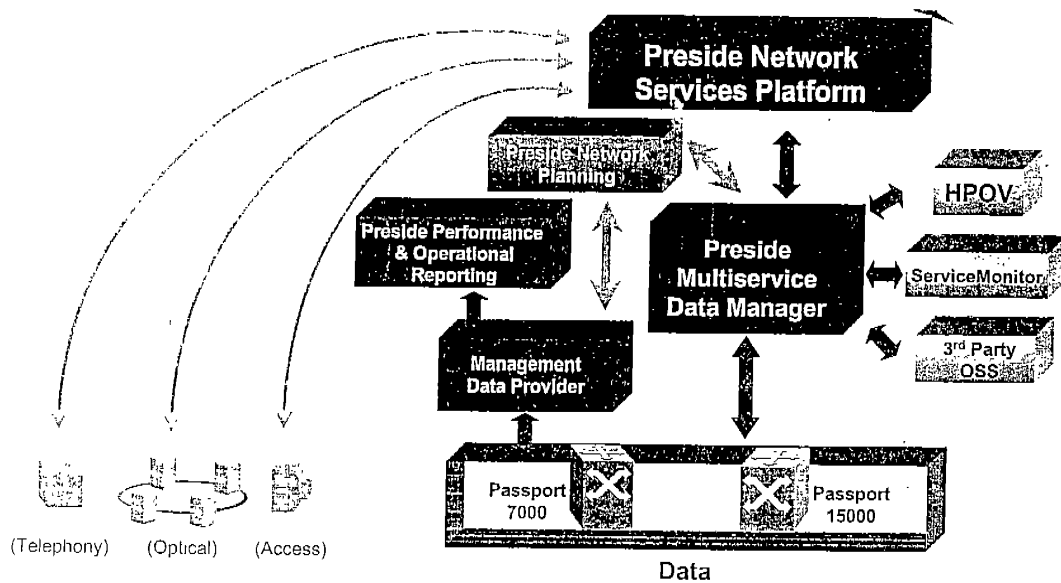
圖 2.3 網路管理設計系統
