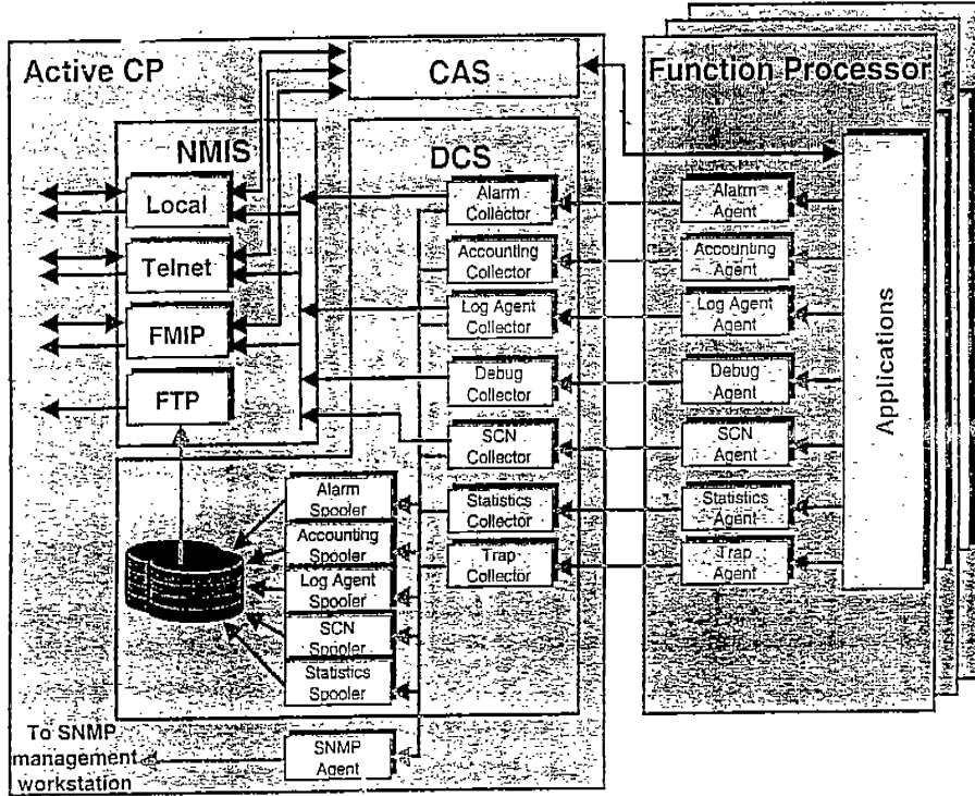
圖 2.2.3-2 Passport NMS 系統
