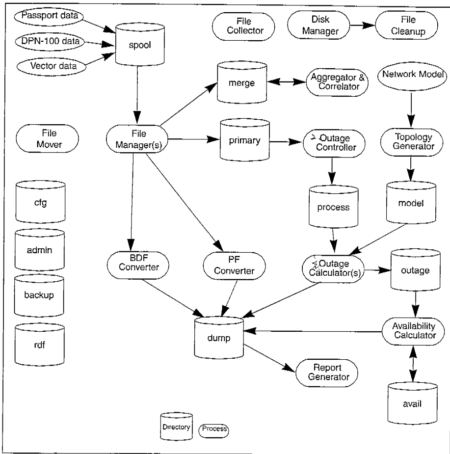
圖 2.3.1.2 MDP 功能處理
